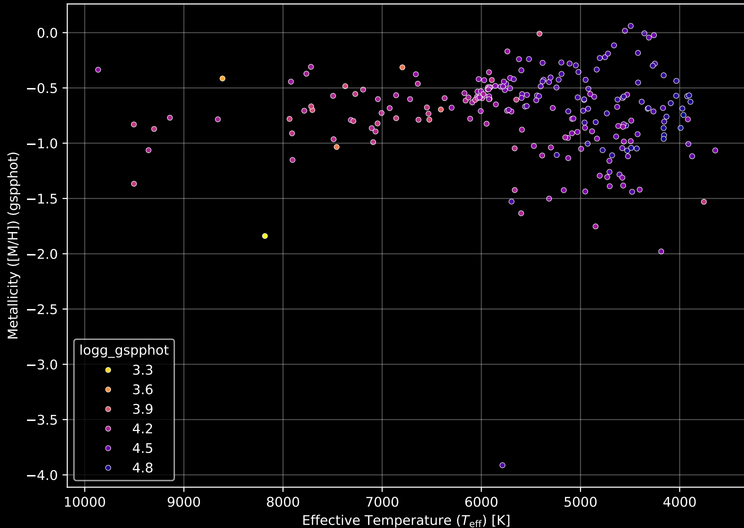
Gaia Cluster: [NGC_2669] Stellar Population Parameters (n= 226)
