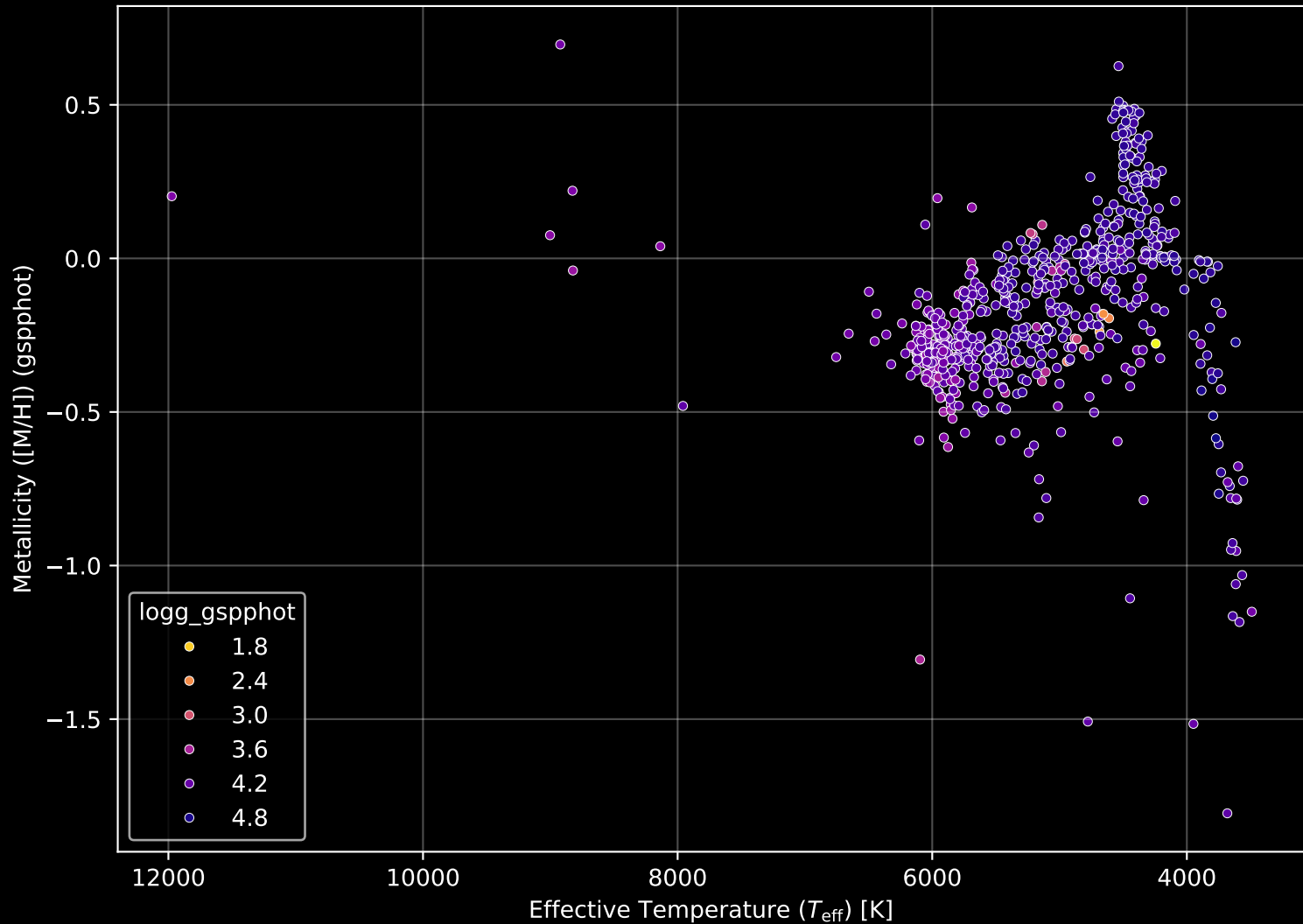
Gaia Cluster: [NGC_2682] Stellar Population Parameters (n= 720)
