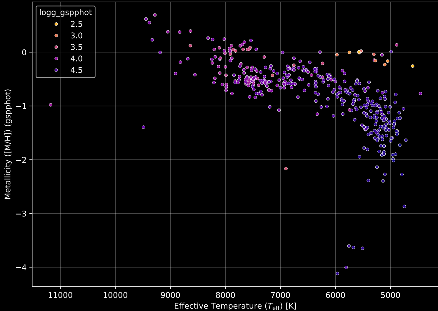
Gaia Cluster: [NGC_2818] Stellar Population Parameters (n= 398)
