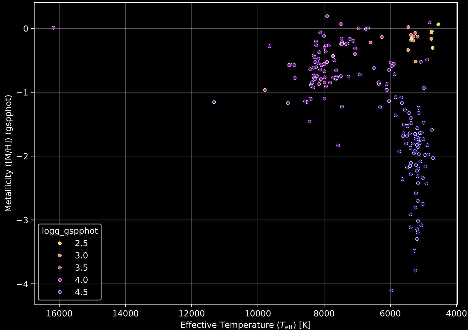
Gaia Cluster: [NGC_2849] Stellar Population Parameters (n= 197)
