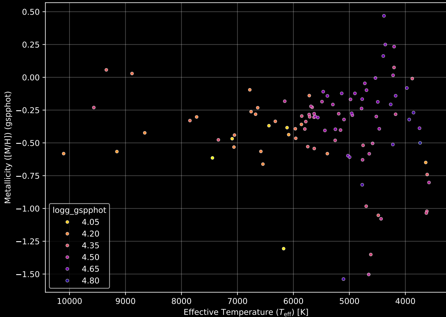
Gaia Cluster: [NGC_2925] Stellar Population Parameters (n= 100)
