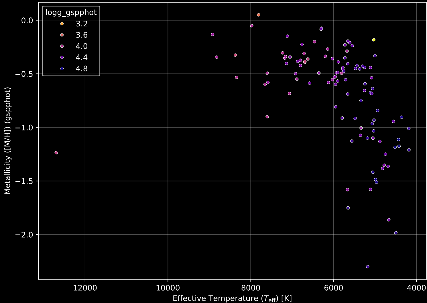
Gaia Cluster: [NGC_3033] Stellar Population Parameters (n= 106)
