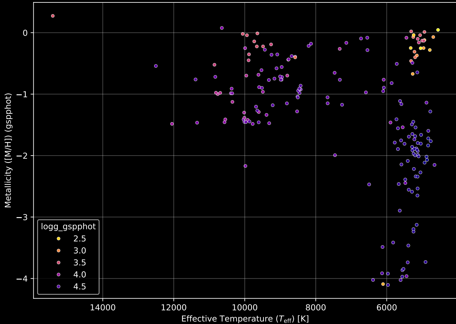
Gaia Cluster: [NGC_3255] Stellar Population Parameters (n= 193)
