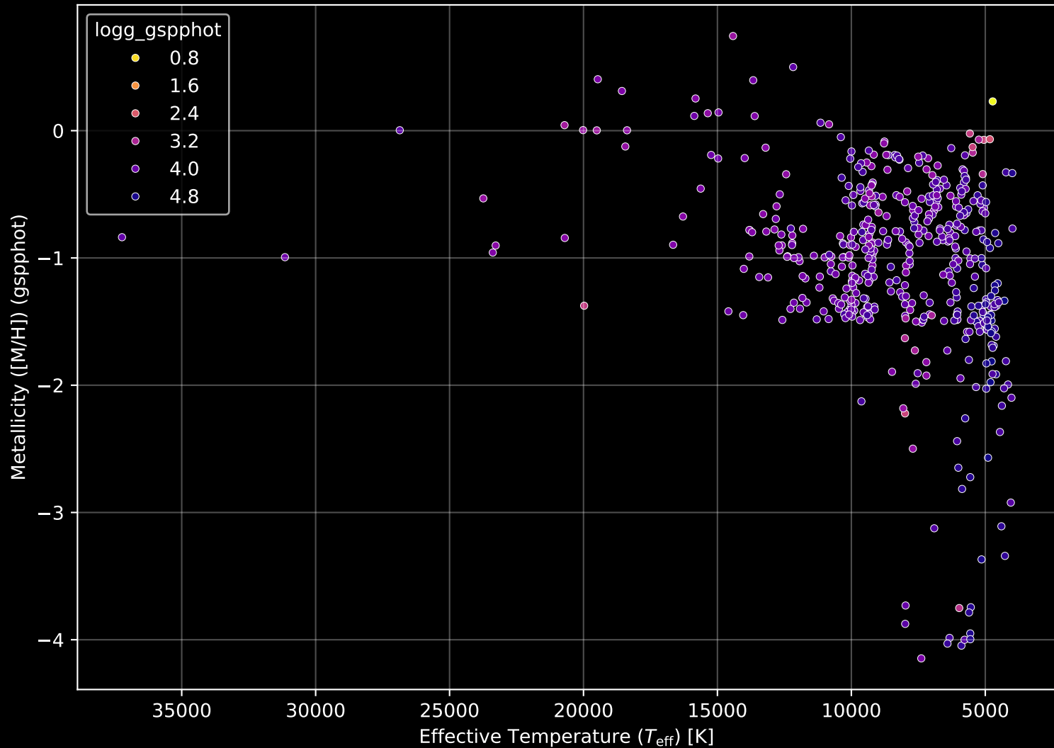
Gaia Cluster: [NGC_3293] Stellar Population Parameters (n= 490)
