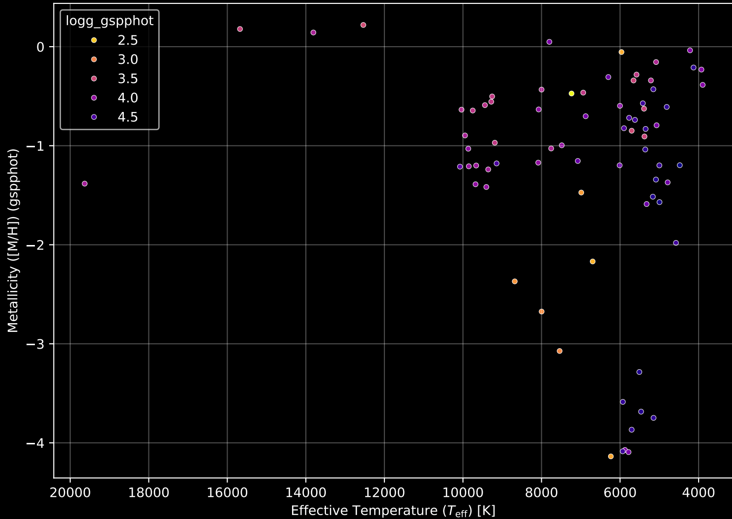
Gaia Cluster: [NGC_3324] Stellar Population Parameters (n= 75)
