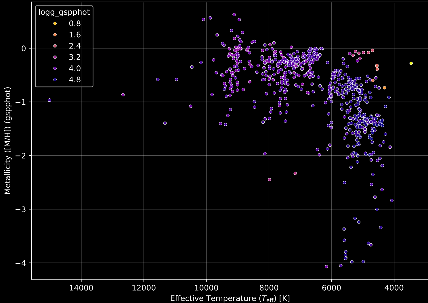
Gaia Cluster: [NGC_3496] Stellar Population Parameters (n= 629)
