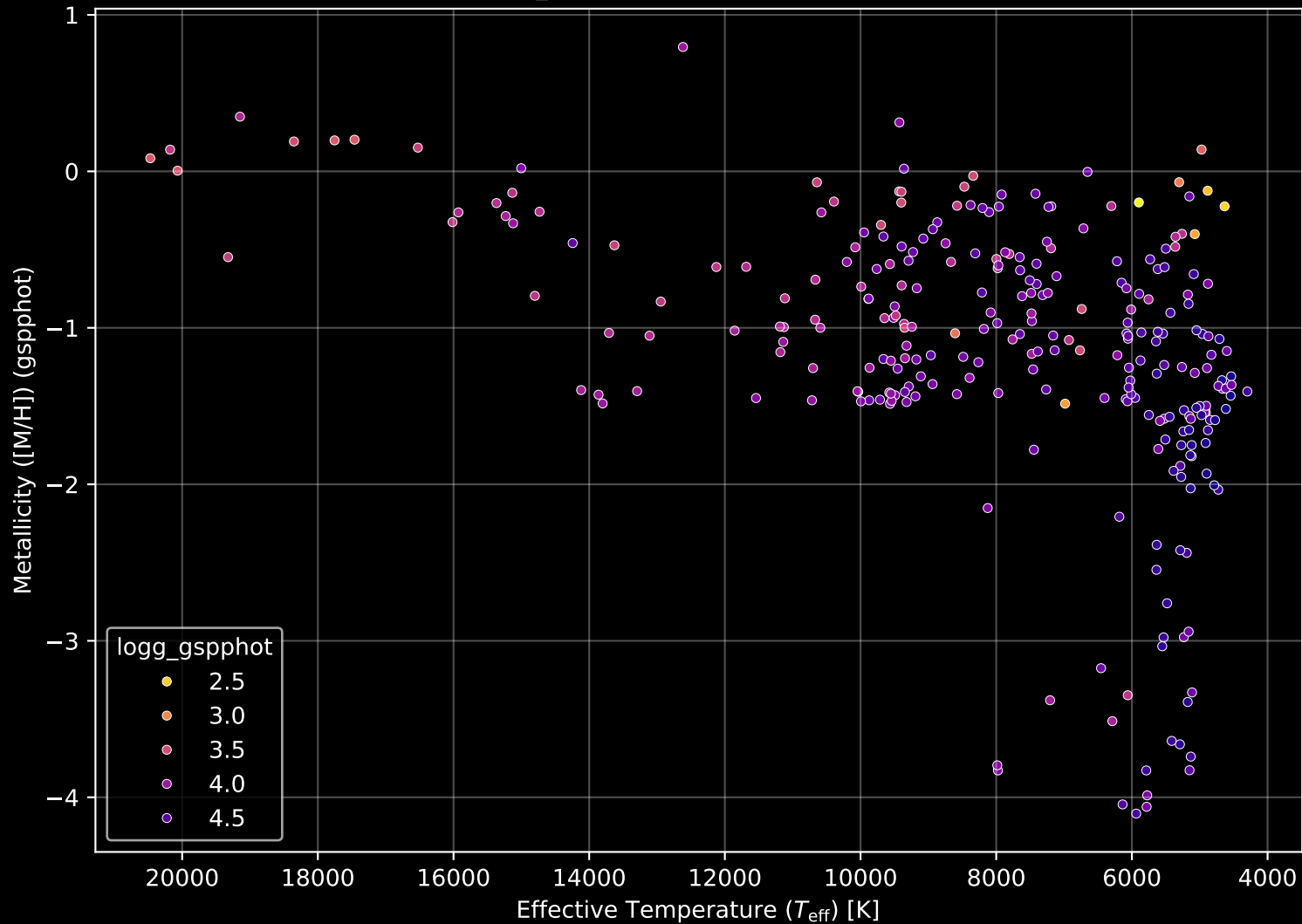
Gaia Cluster: [NGC_3590] Stellar Population Parameters (n= 282)
