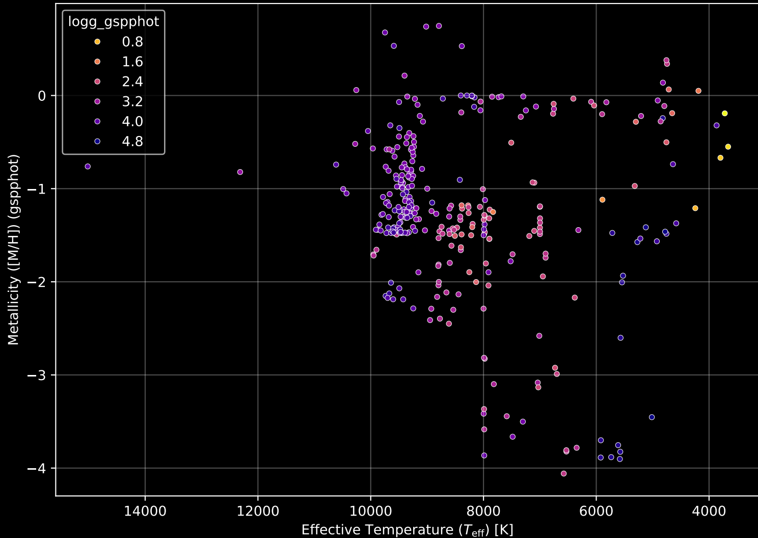
Gaia Cluster: [NGC_3603] Stellar Population Parameters (n= 327)
