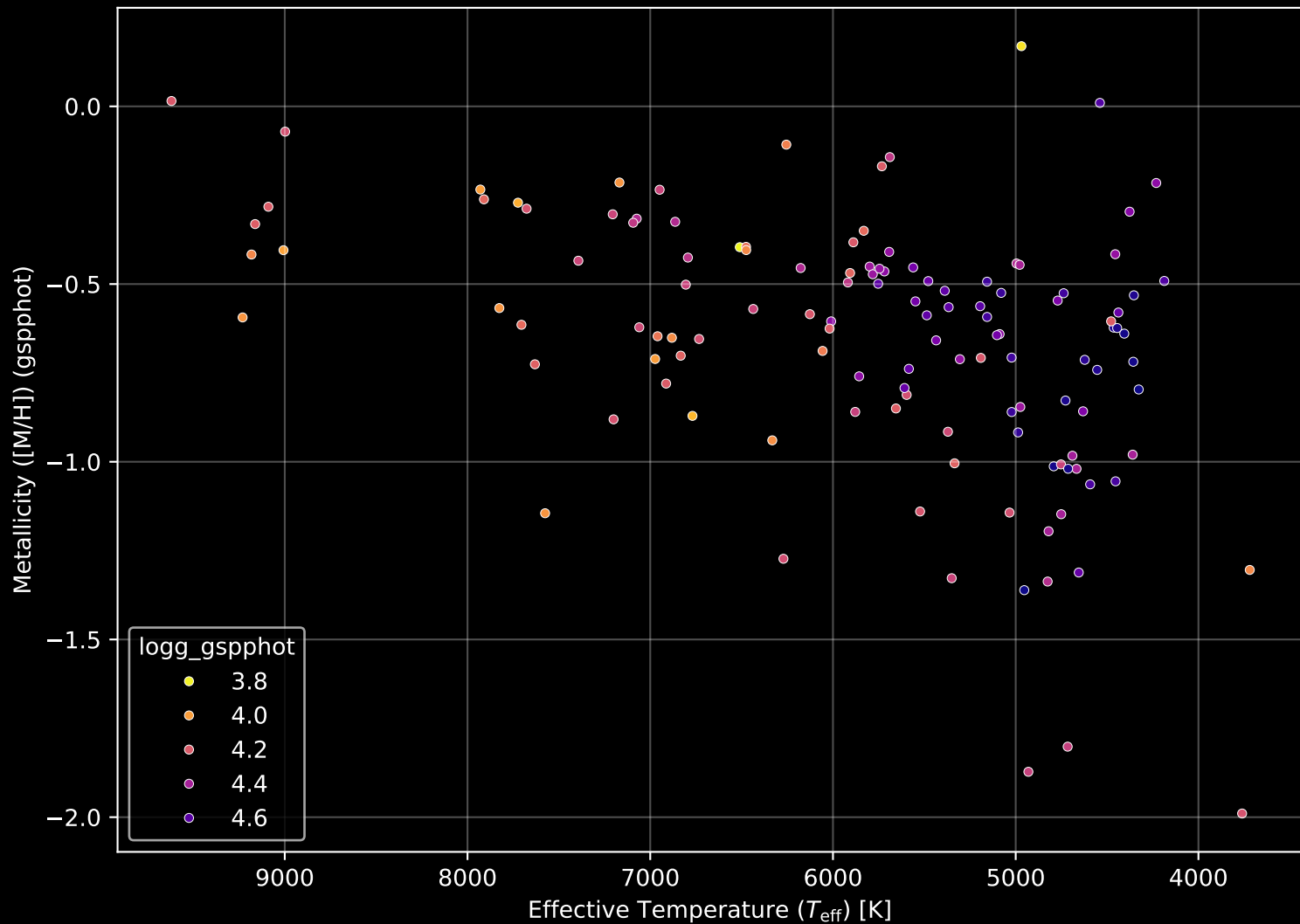
Gaia Cluster: [NGC_381] Stellar Population Parameters (n= 126)
