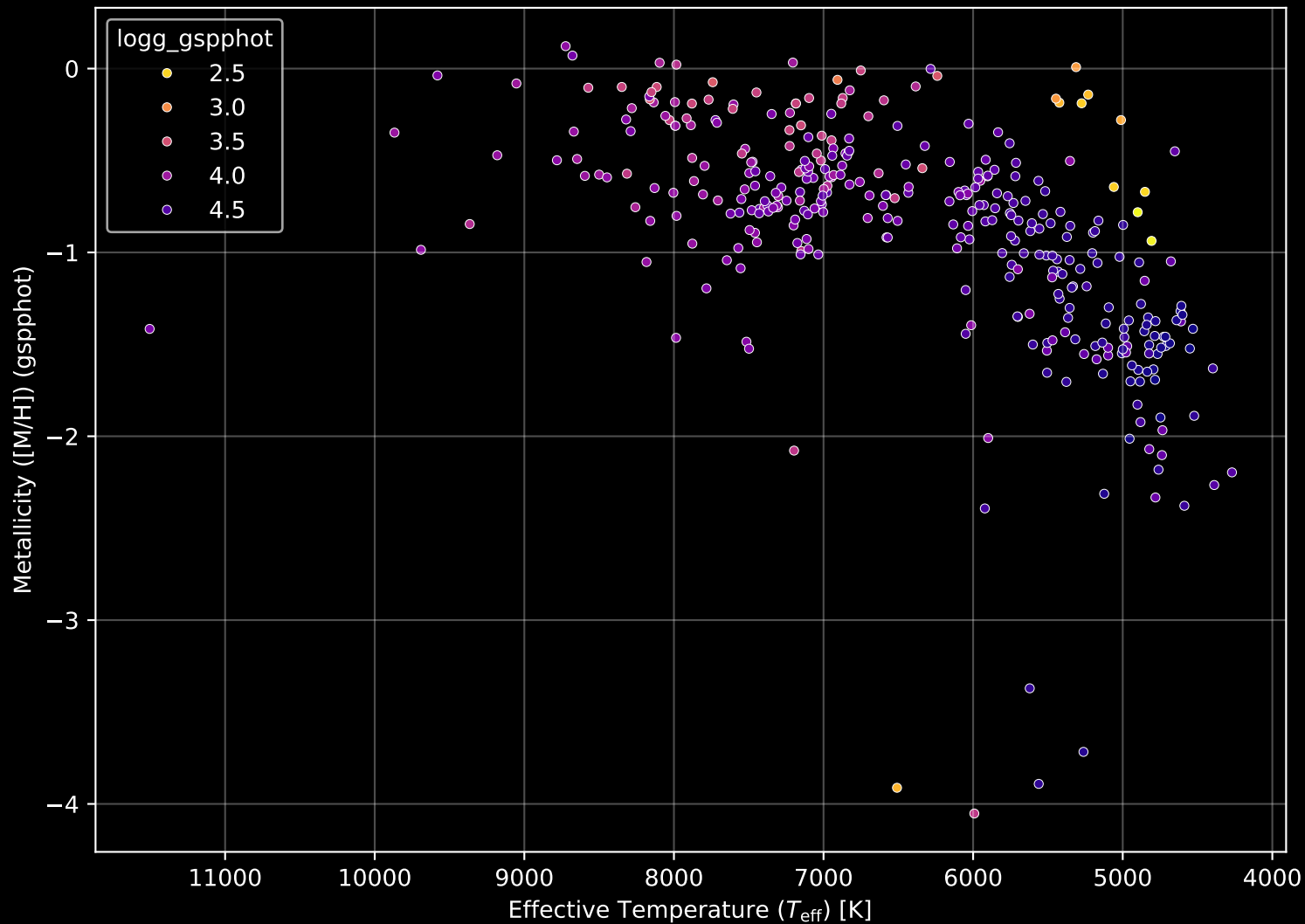
Gaia Cluster: [NGC_3960] Stellar Population Parameters (n= 352)
