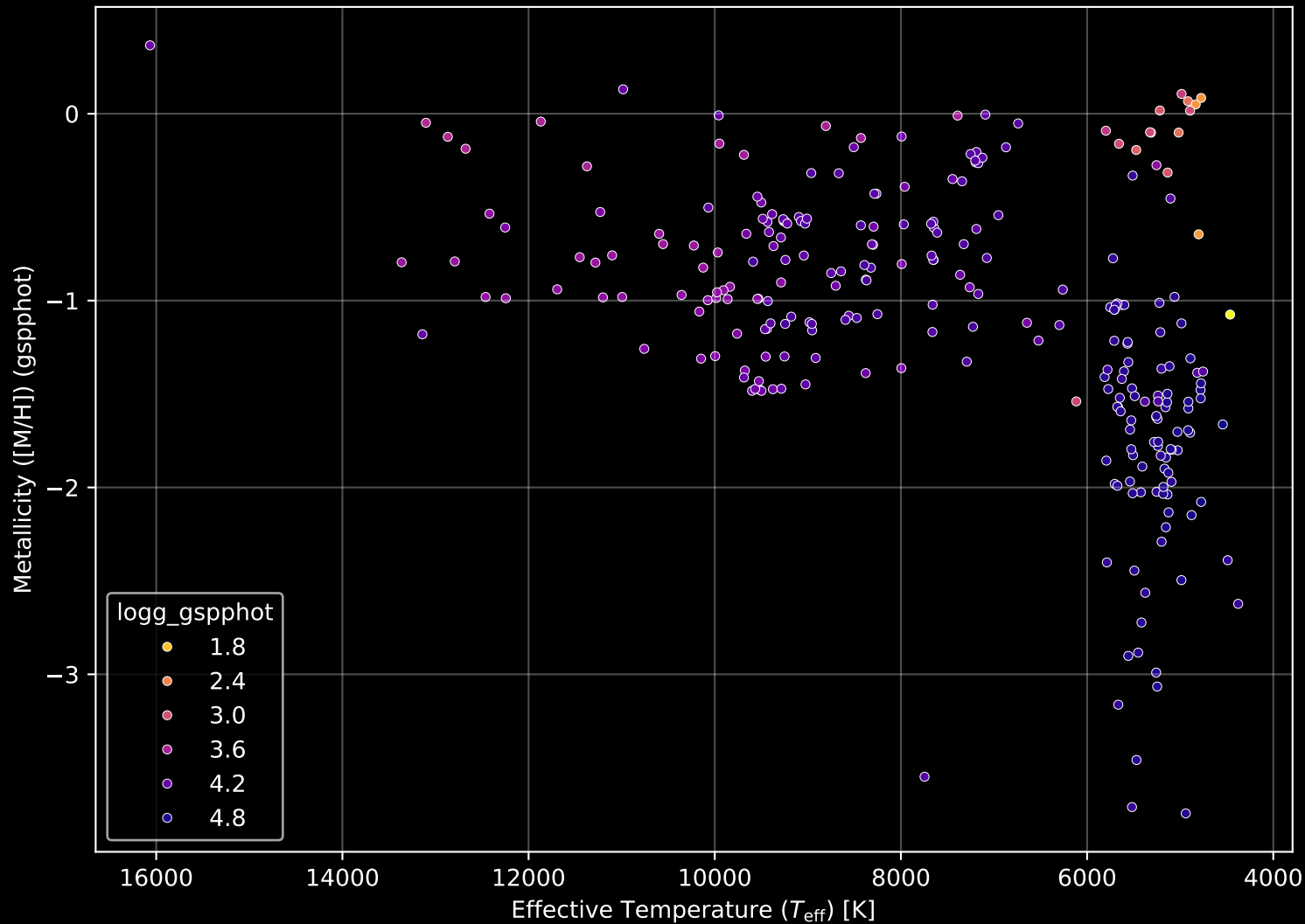
Gaia Cluster: [NGC_436] Stellar Population Parameters (n= 265)
