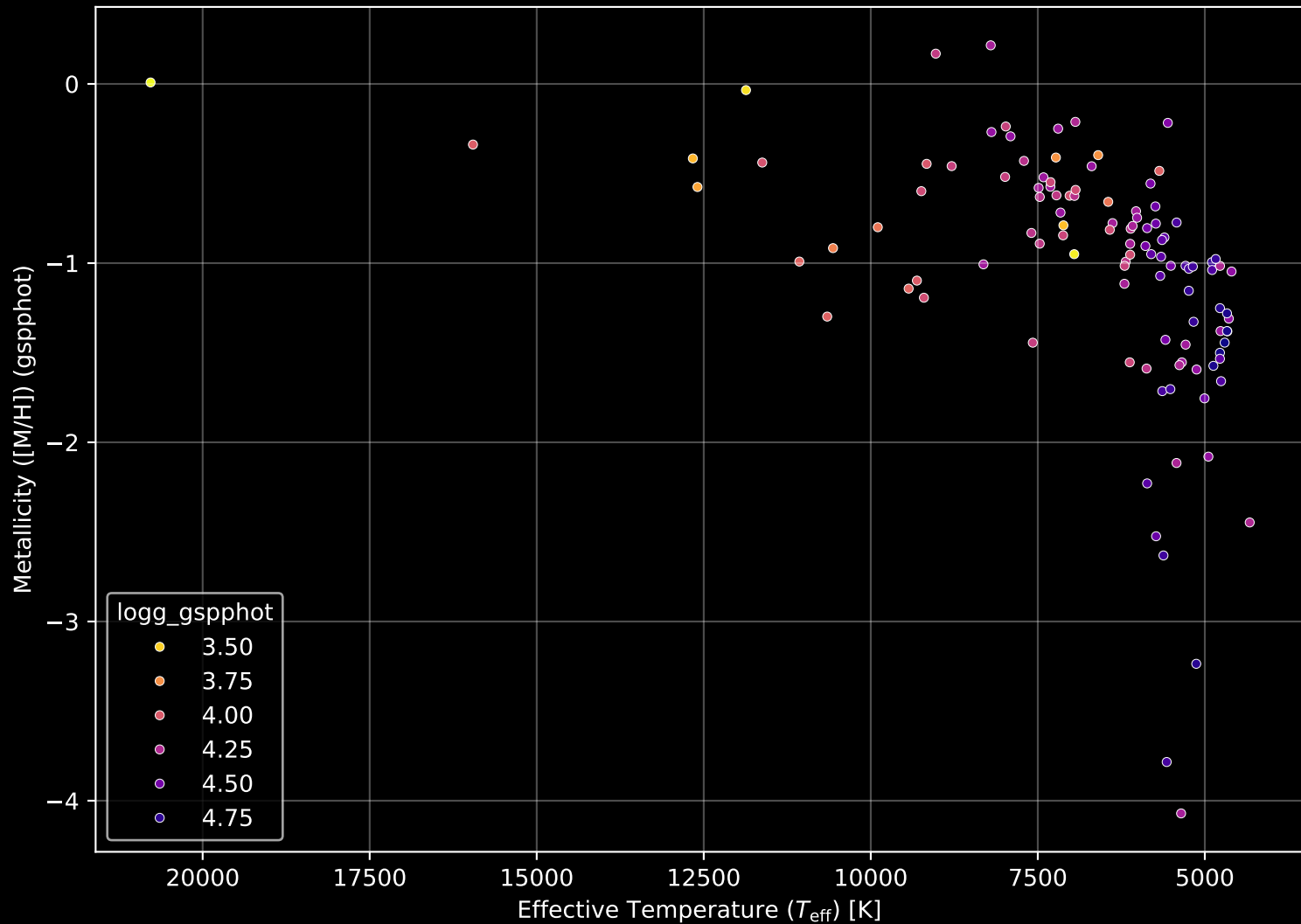
Gaia Cluster: [NGC_4463] Stellar Population Parameters (n= 111)
