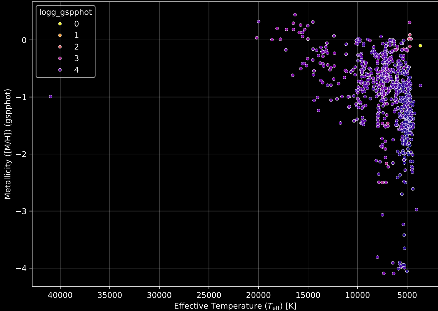
Gaia Cluster: [NGC_4755] Stellar Population Parameters (n= 834)
