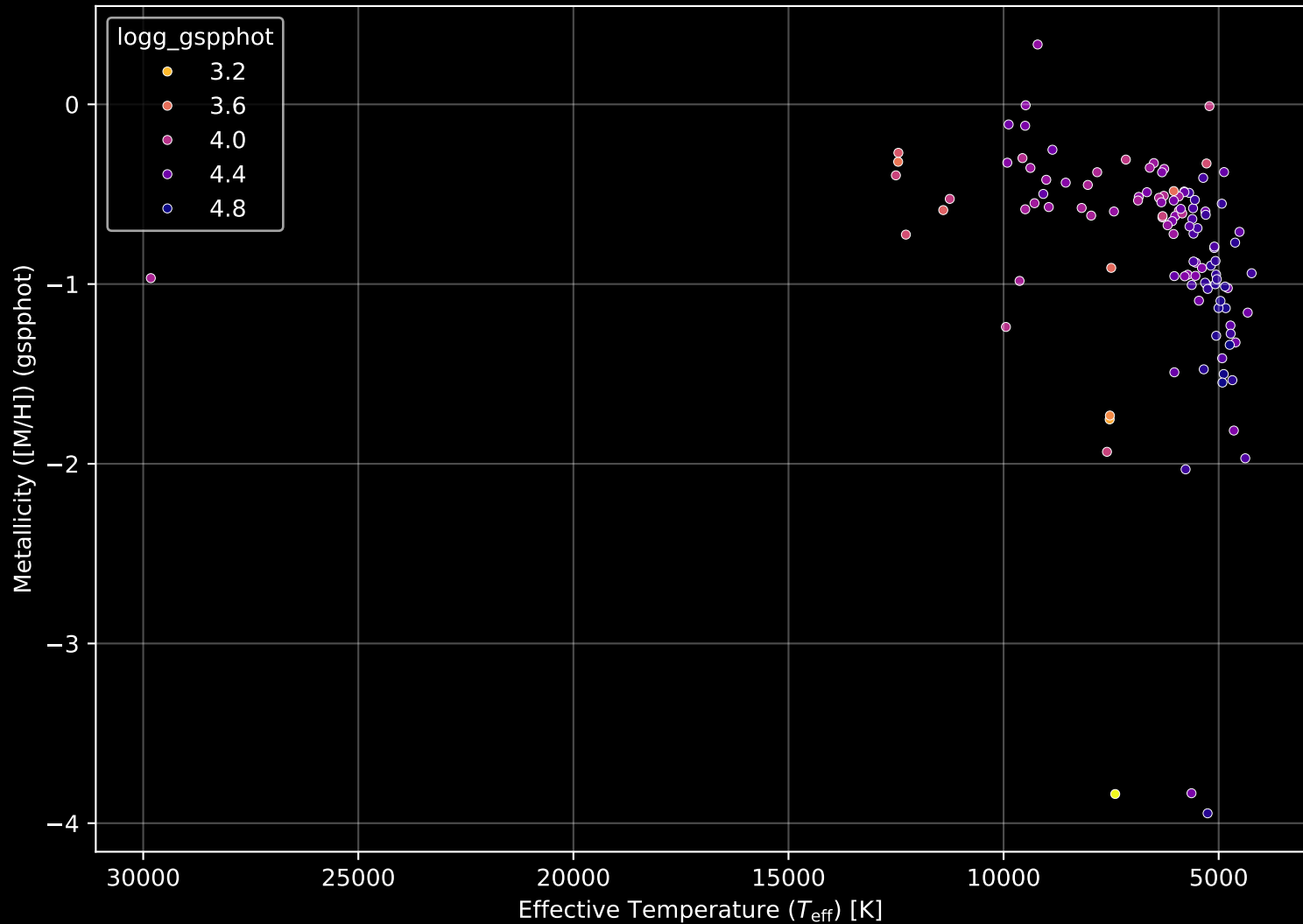
Gaia Cluster: [NGC_5281] Stellar Population Parameters (n= 116)
