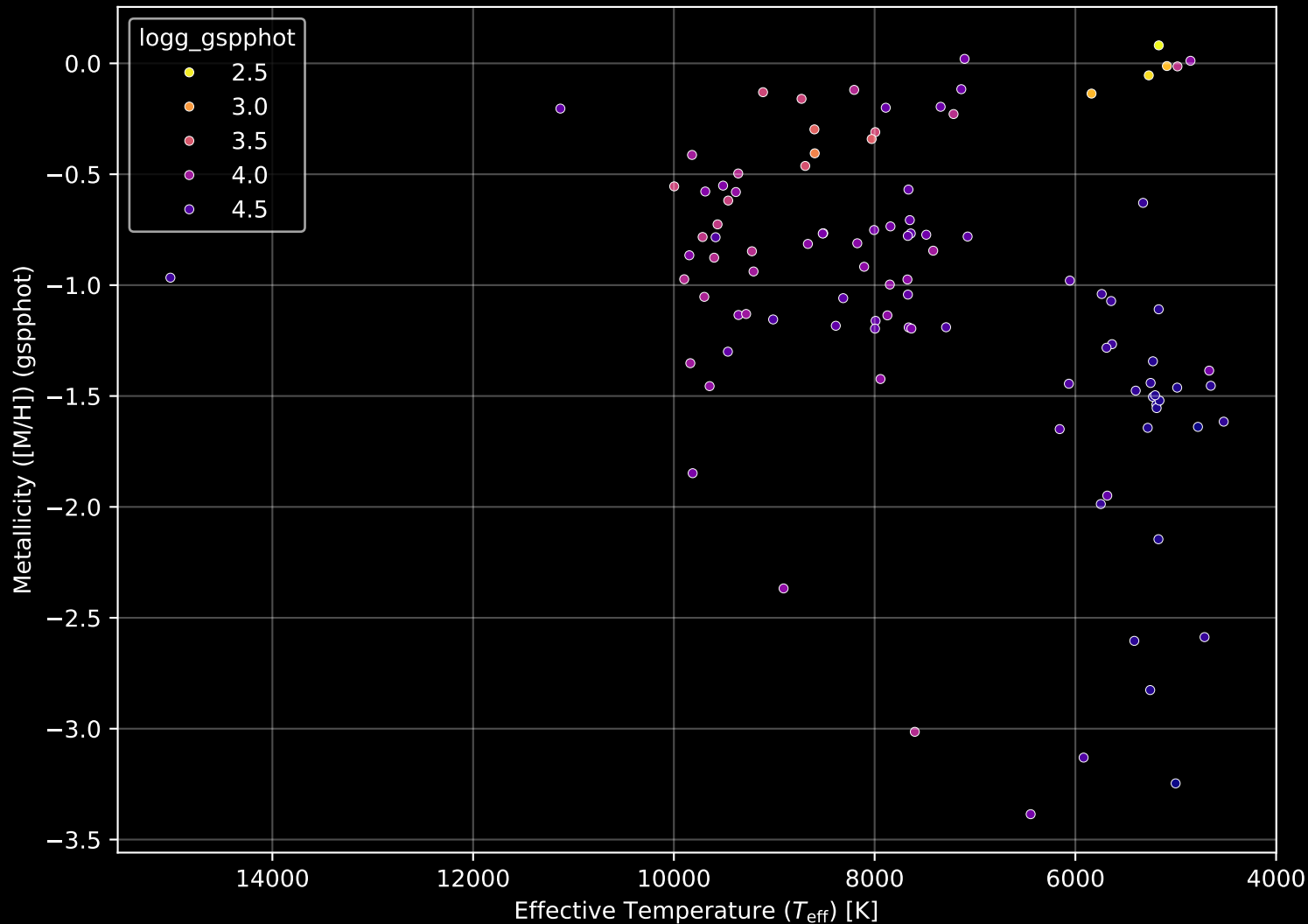
Gaia Cluster: [NGC_5288] Stellar Population Parameters (n= 104)
