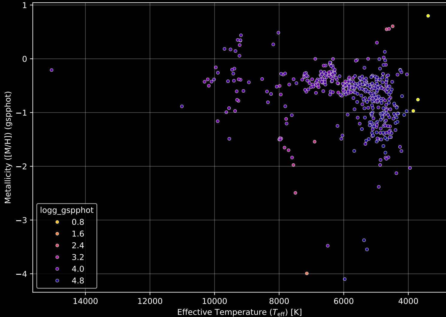
Gaia Cluster: [NGC_5316] Stellar Population Parameters (n= 457)
