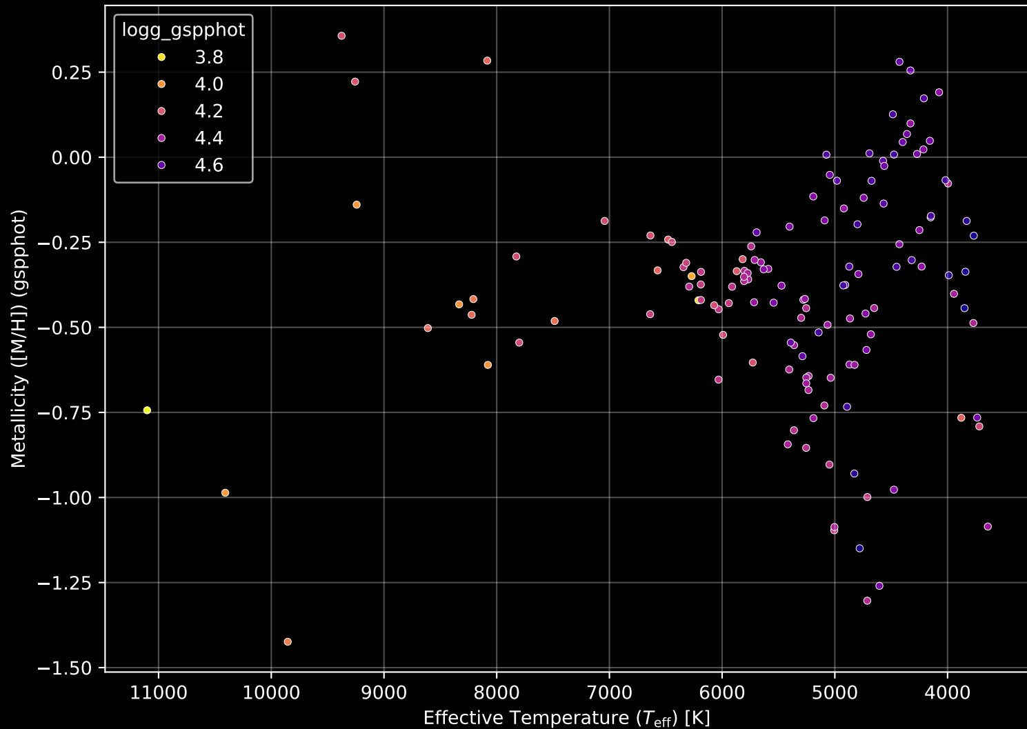
Gaia Cluster: [NGC_5460] Stellar Population Parameters (n= 139)
