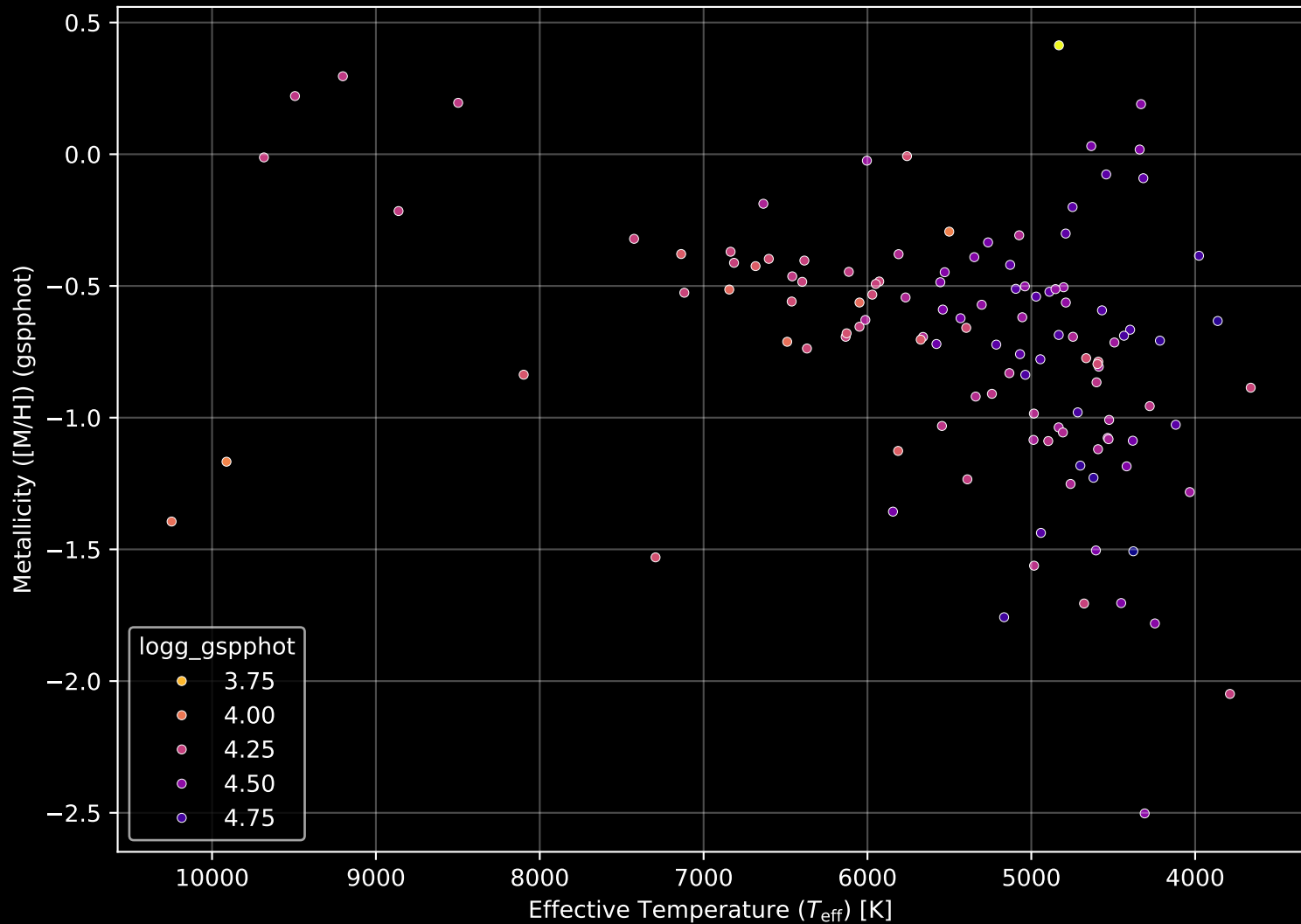
Gaia Cluster: [NGC_5593] Stellar Population Parameters (n= 121)
