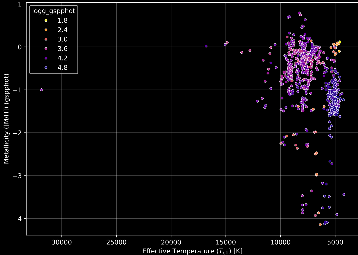
Gaia Cluster: [NGC_5617] Stellar Population Parameters (n= 816)
