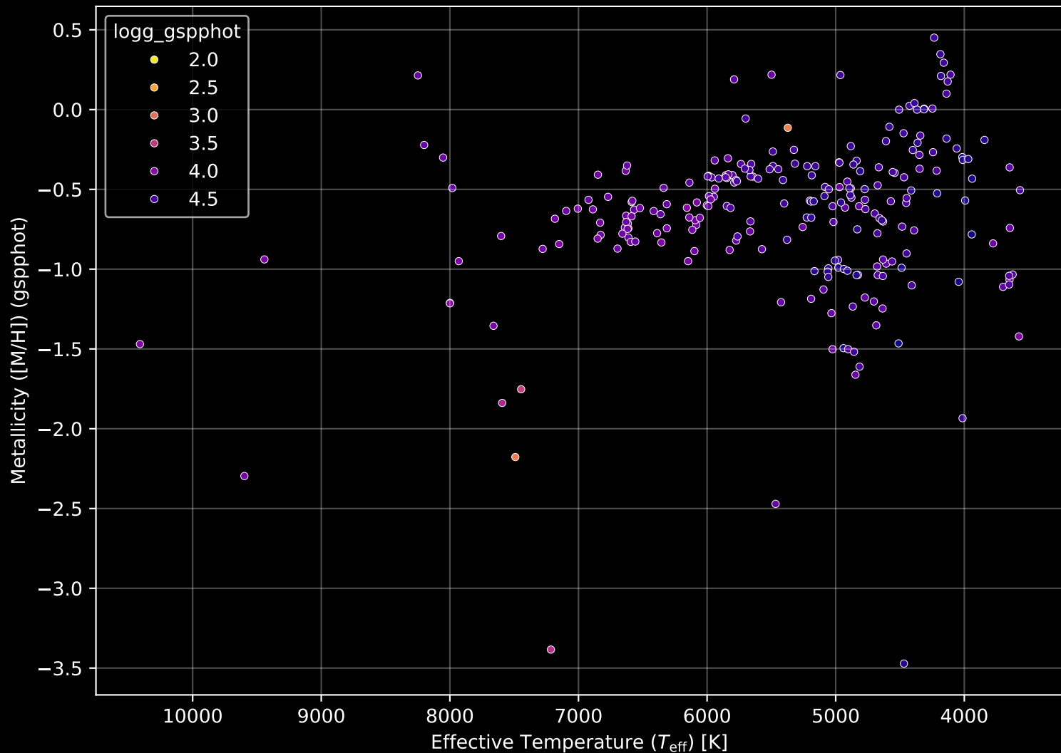
Gaia Cluster: [NGC_5662] Stellar Population Parameters (n= 245)
