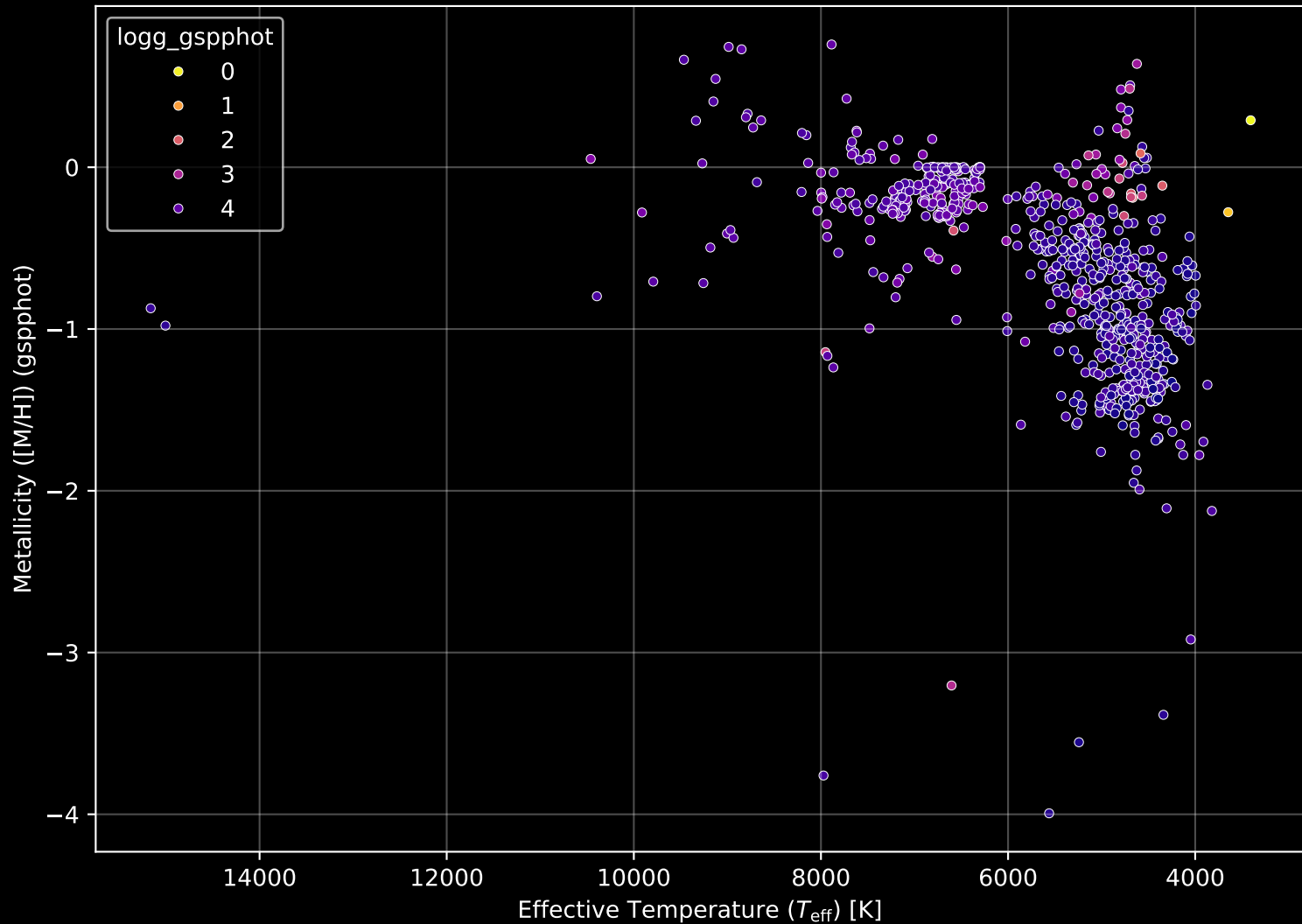
Gaia Cluster: [NGC_5925] Stellar Population Parameters (n= 769)
