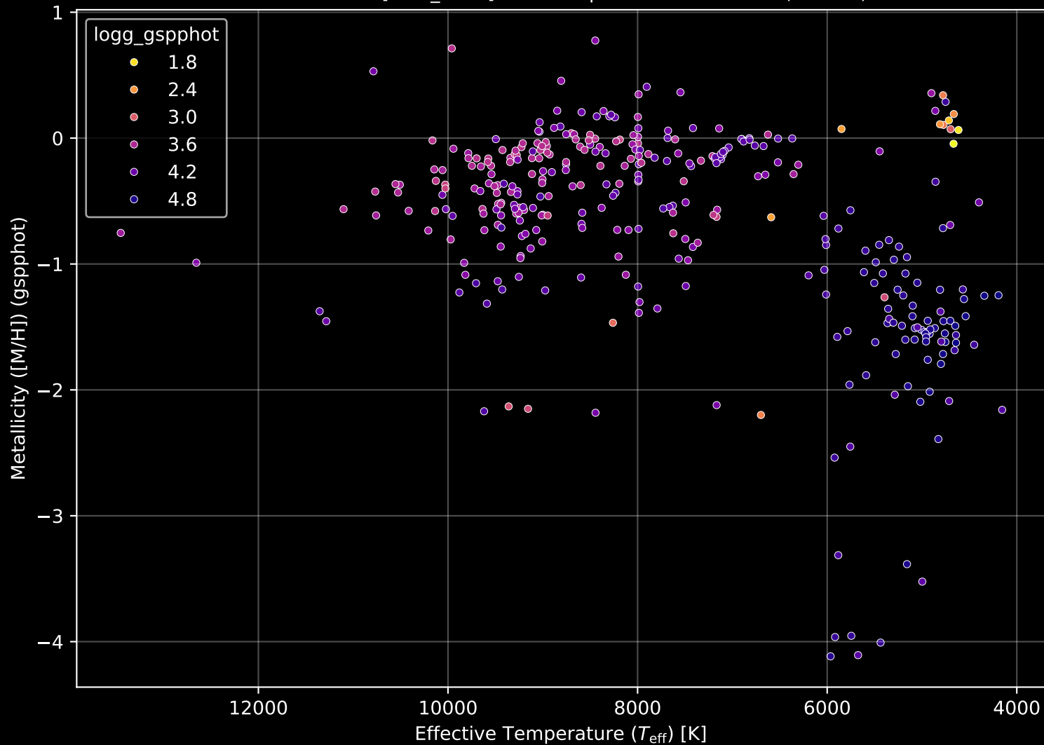
Gaia Cluster: [NGC_5999] Stellar Population Parameters (n= 358)
