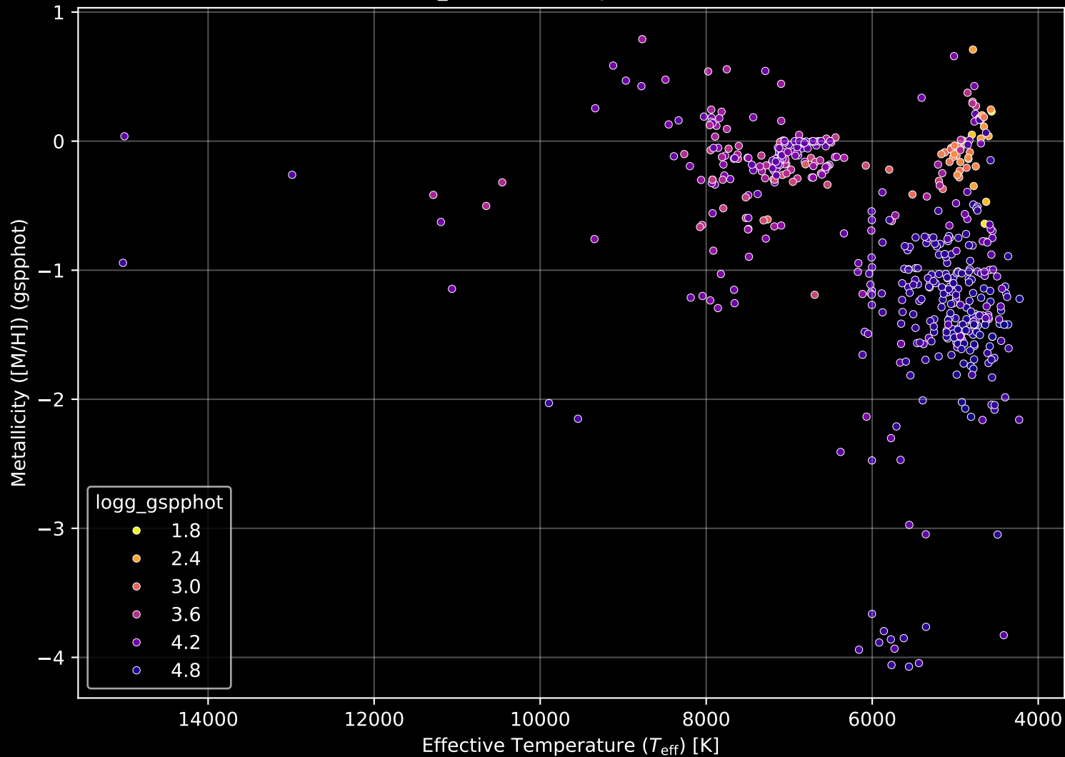
Gaia Cluster: [NGC_6005] Stellar Population Parameters (n= 542)
