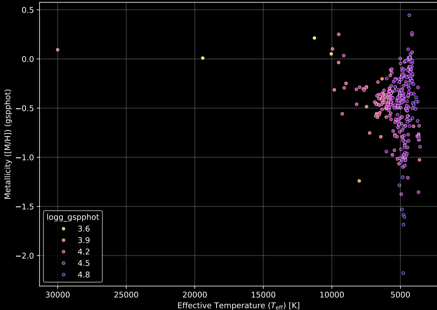
Gaia Cluster: [NGC_6025] Stellar Population Parameters (n= 307)
