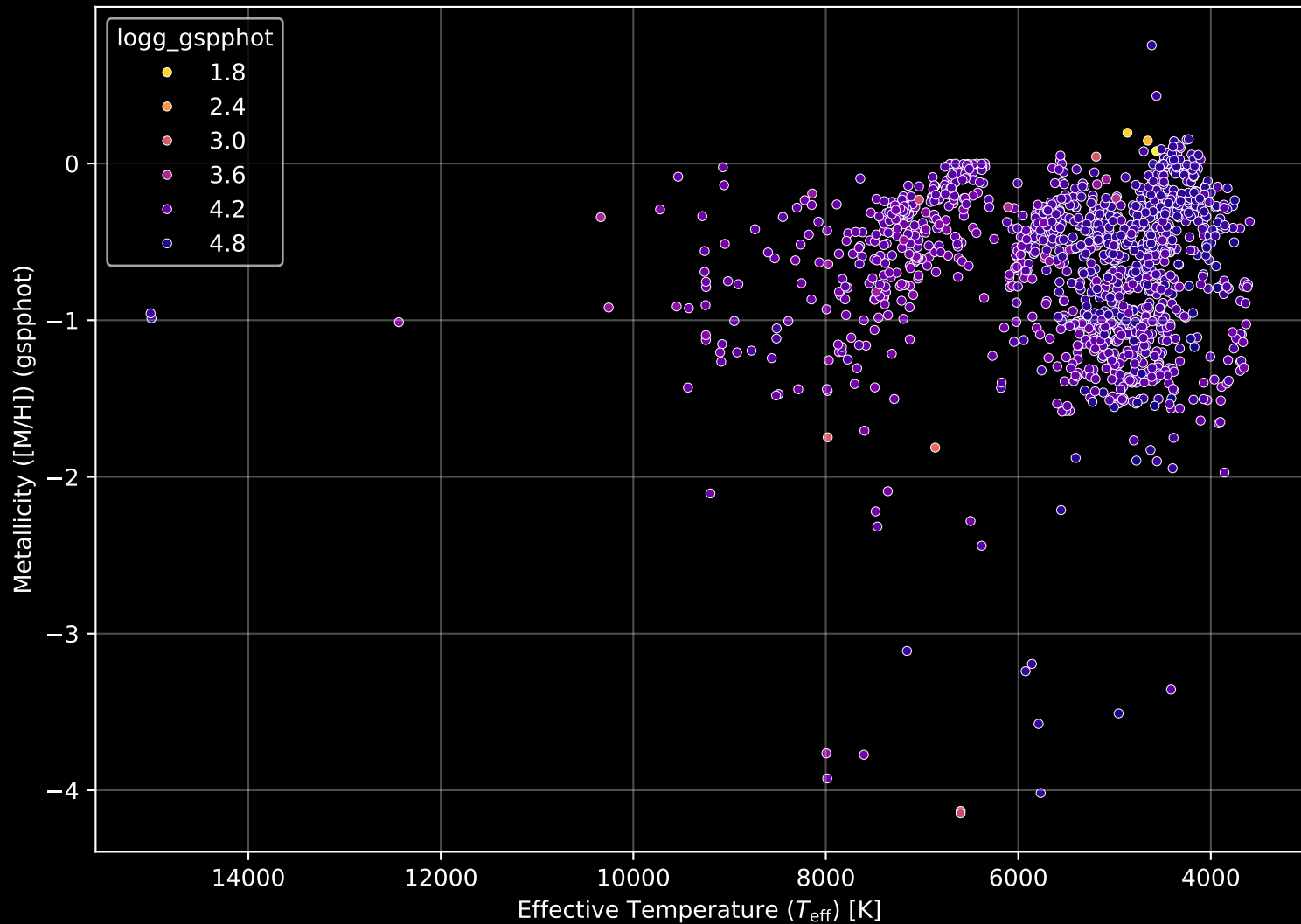
Gaia Cluster: [NGC_6124] Stellar Population Parameters (n= 1259)
