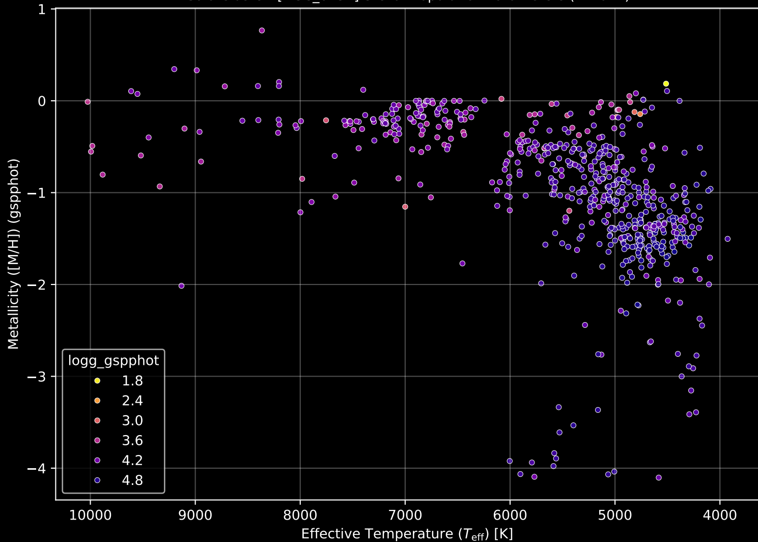
Gaia Cluster: [NGC_6152] Stellar Population Parameters (n= 622)
