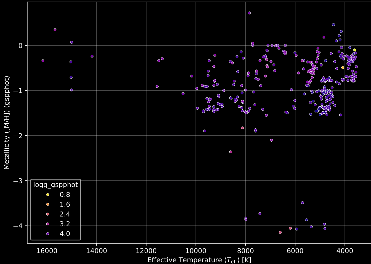
Gaia Cluster: [NGC_6193] Stellar Population Parameters (n= 359)
