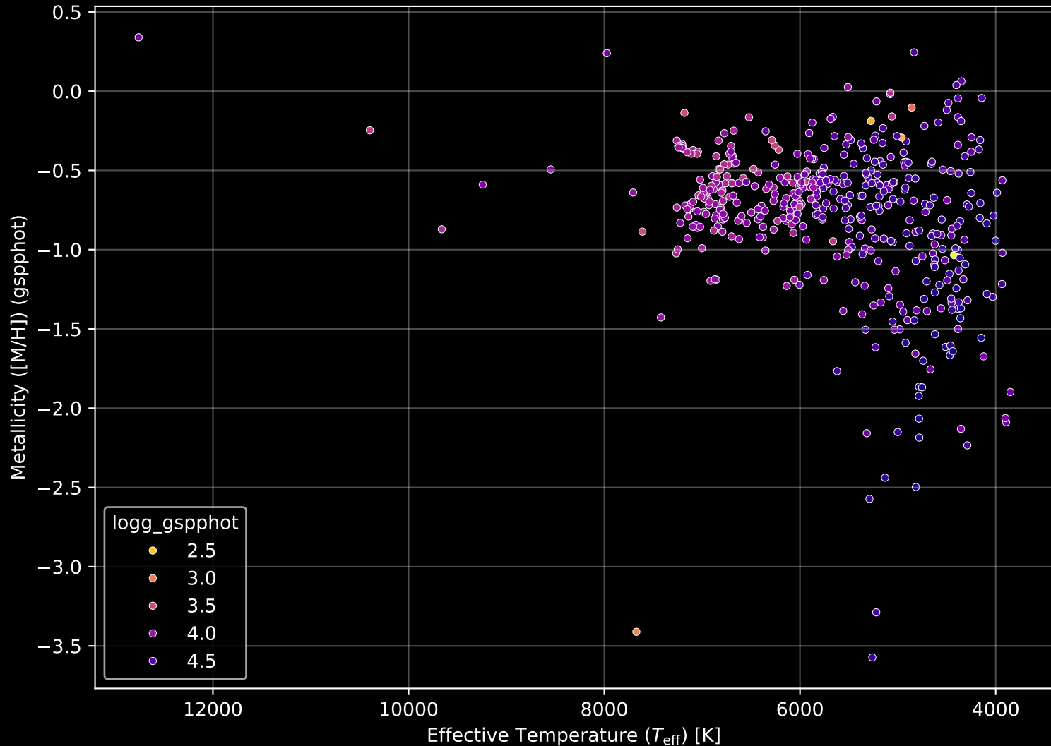
Gaia Cluster: [NGC_6208] Stellar Population Parameters (n= 455)
