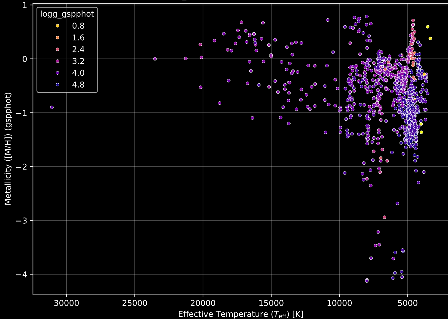
Gaia Cluster: [NGC_6231] Stellar Population Parameters (n= 1080)
