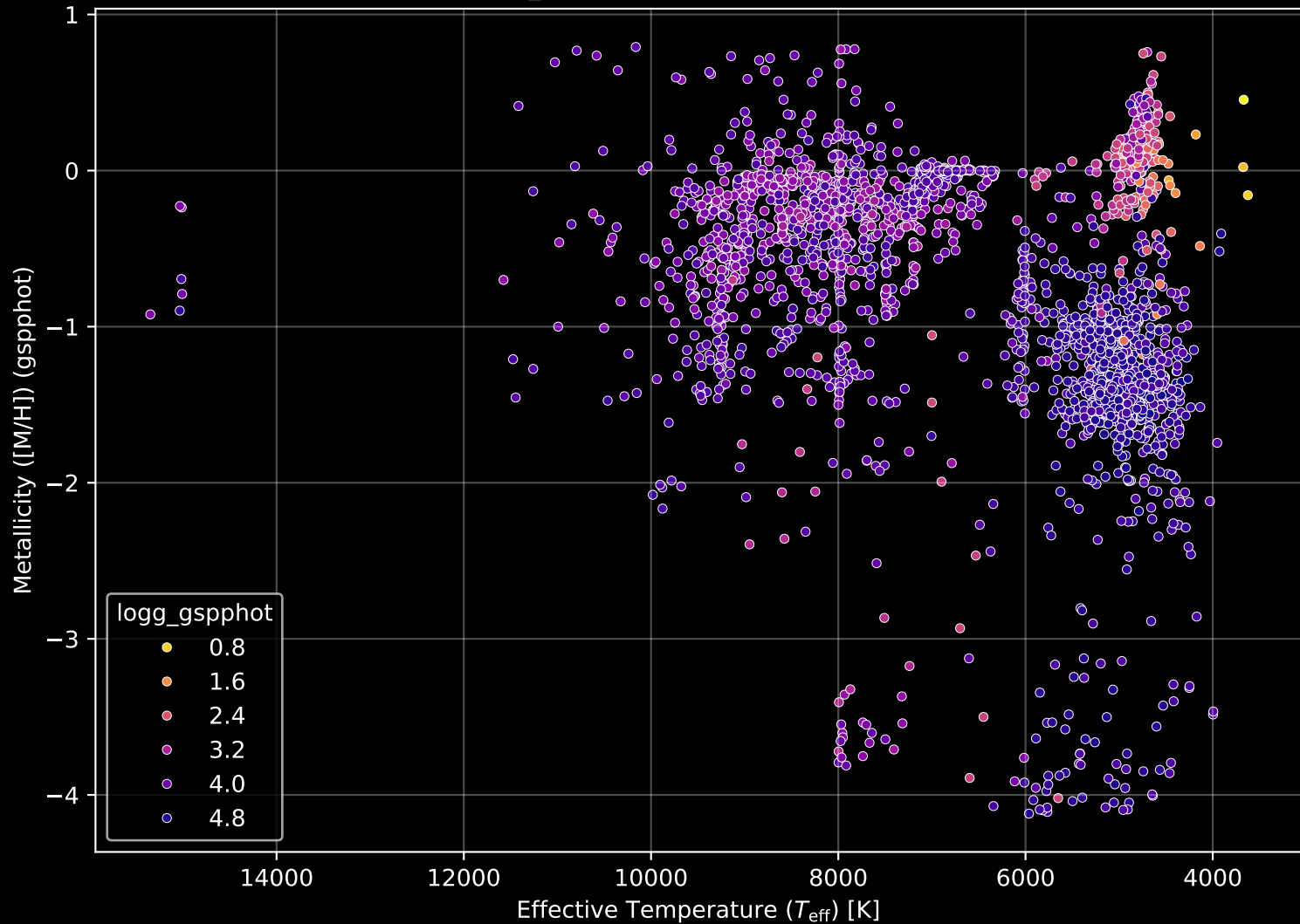
Gaia Cluster: [NGC_6259] Stellar Population Parameters (n= 2578)
