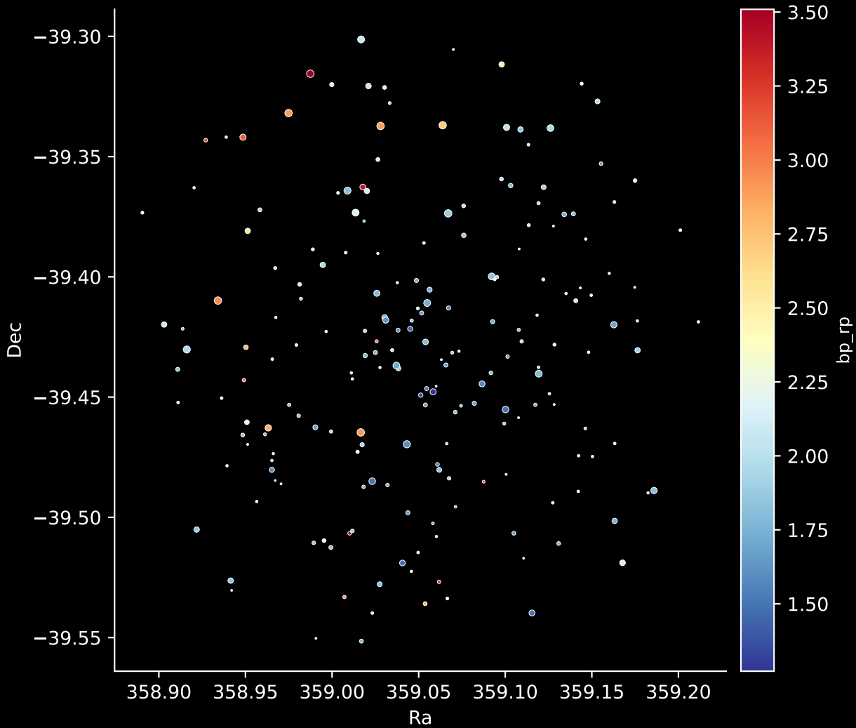
Gaia Cluster: [NGC_6318] Stars: 202
