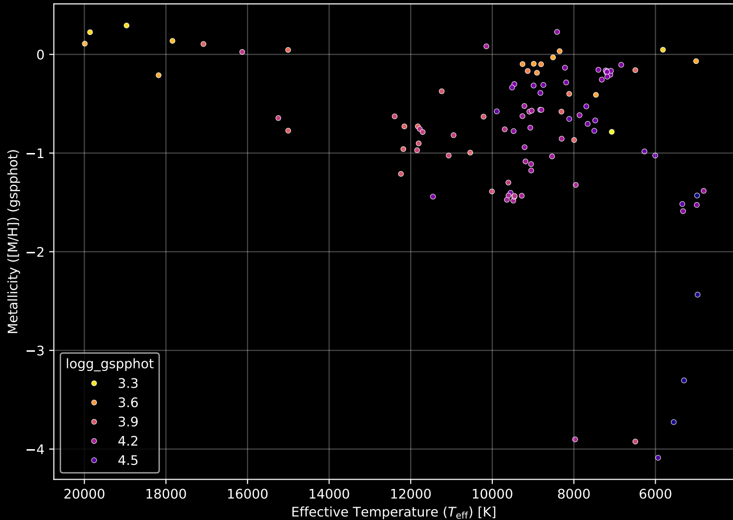
Gaia Cluster: [NGC_637] Stellar Population Parameters (n= 104)
