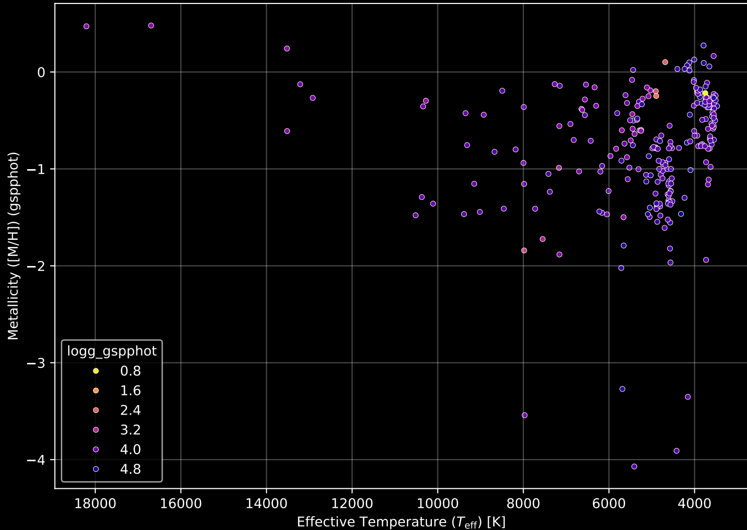
Gaia Cluster: [NGC_6383] Stellar Population Parameters (n= 271)
