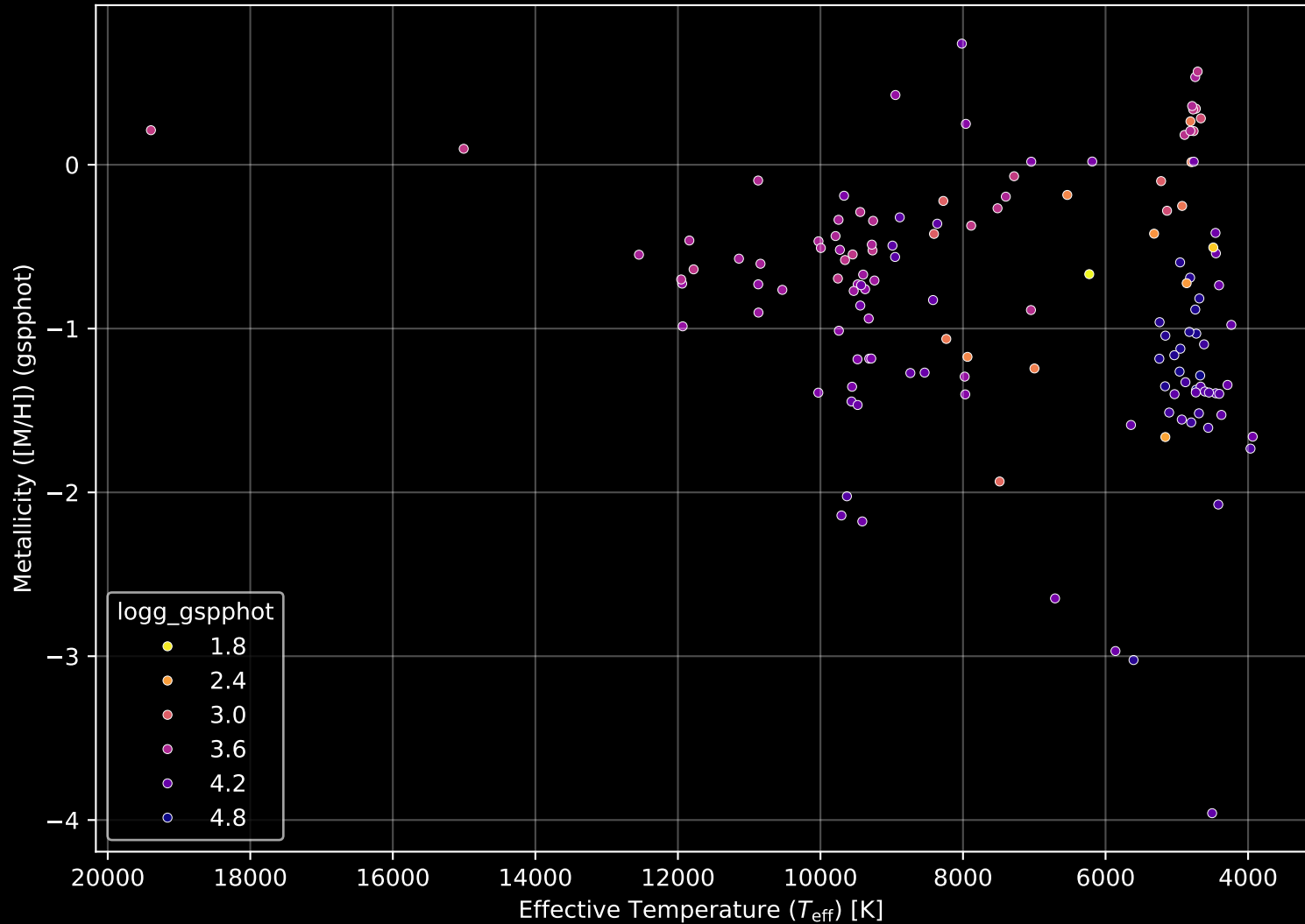
Gaia Cluster: [NGC_6396] Stellar Population Parameters (n= 135)
