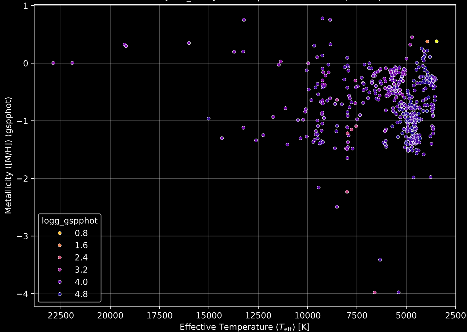
Gaia Cluster: [NGC_6531] Stellar Population Parameters (n= 514)
