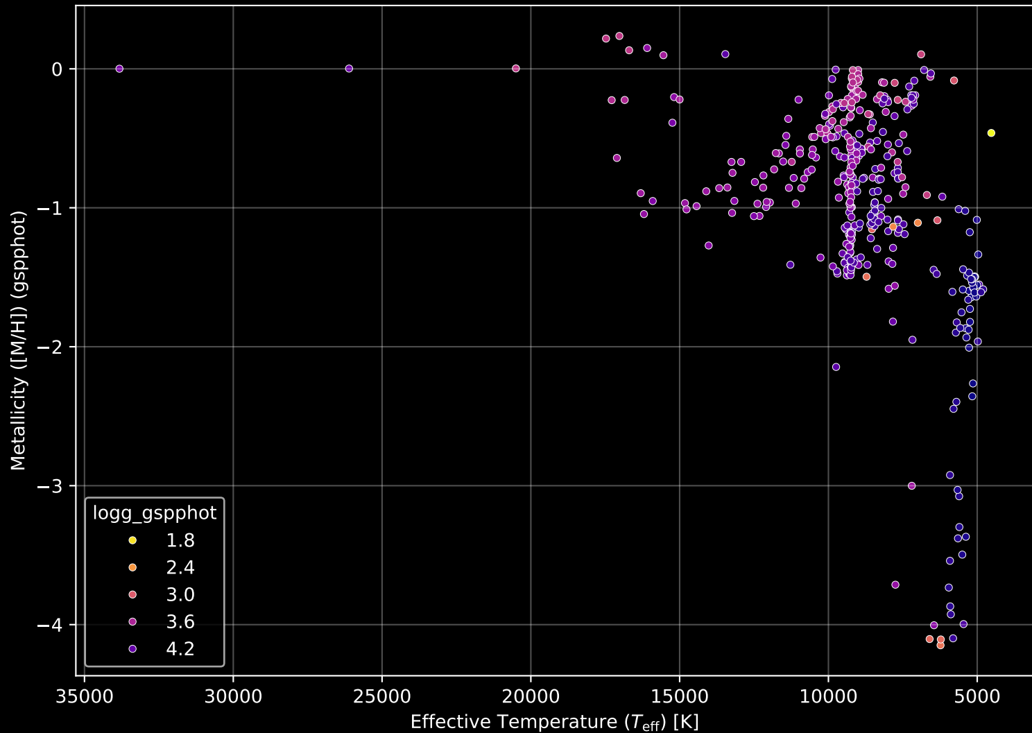
Gaia Cluster: [NGC_654] Stellar Population Parameters (n= 403)
