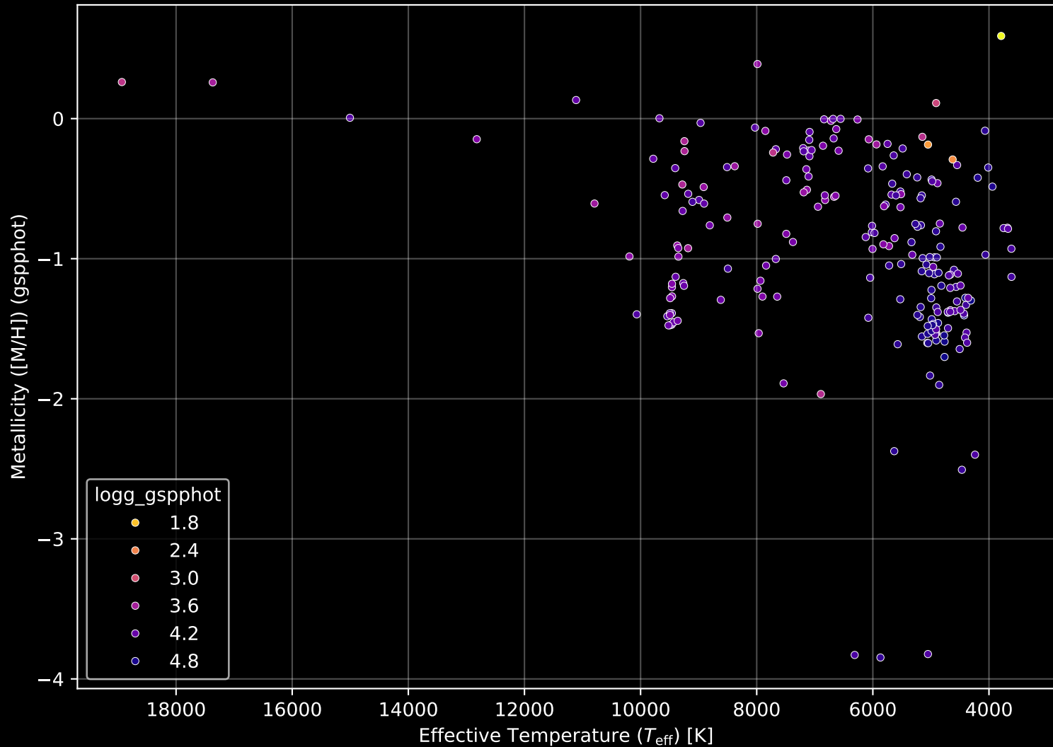
Gaia Cluster: [NGC_6561] Stellar Population Parameters (n= 227)
