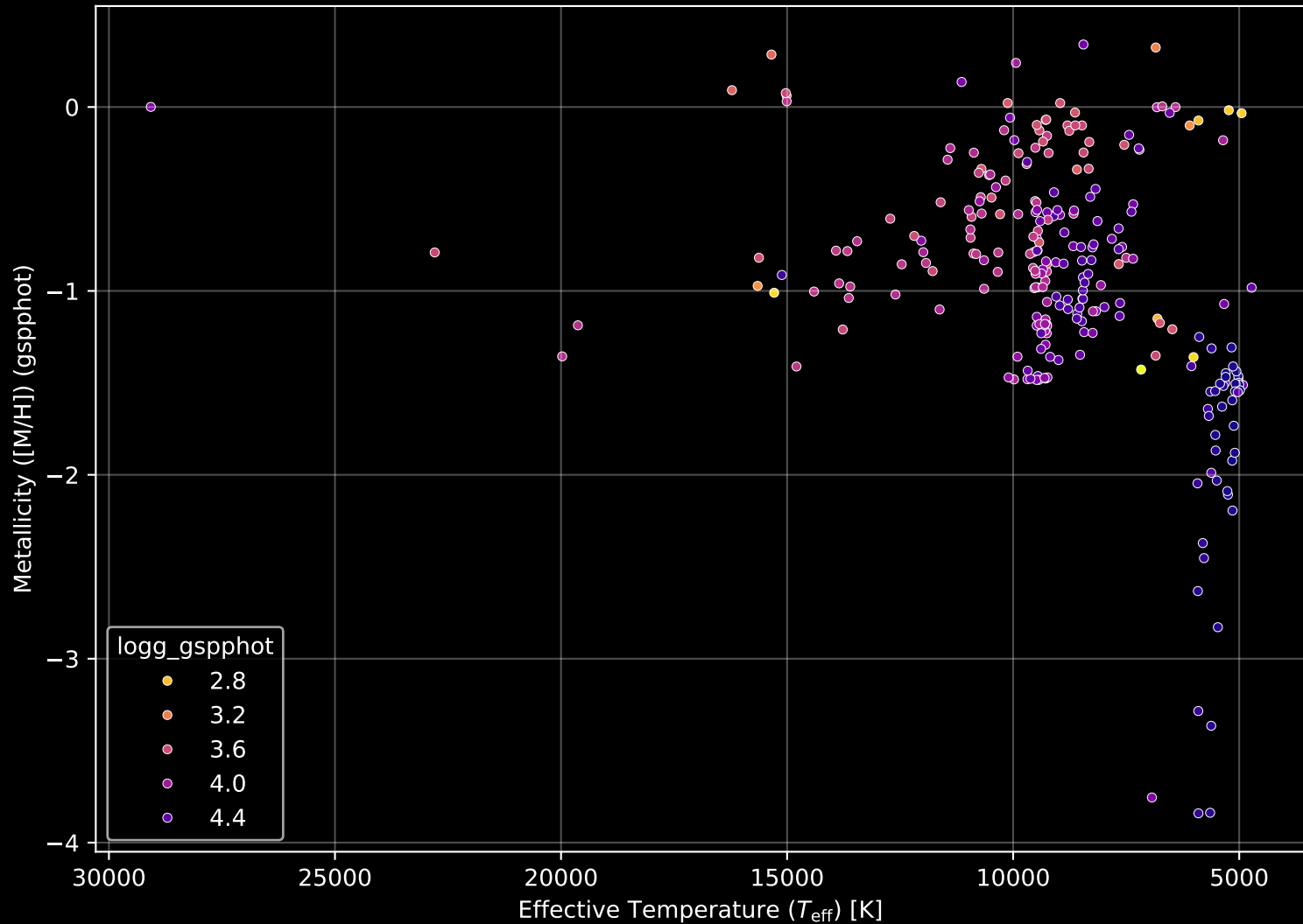
Gaia Cluster: [NGC_659] Stellar Population Parameters (n= 262)
