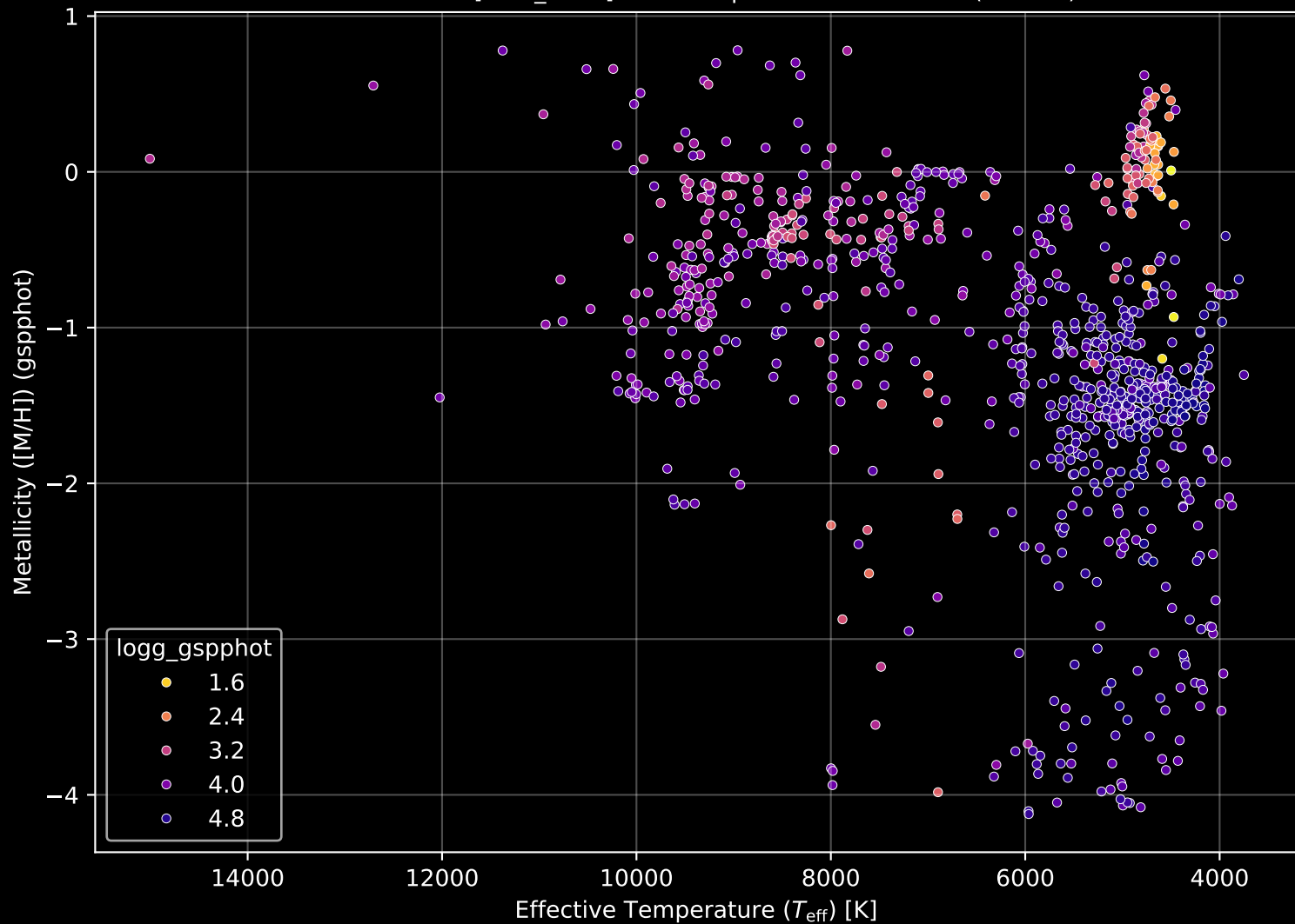
Gaia Cluster: [NGC_6603] Stellar Population Parameters (n= 948)
