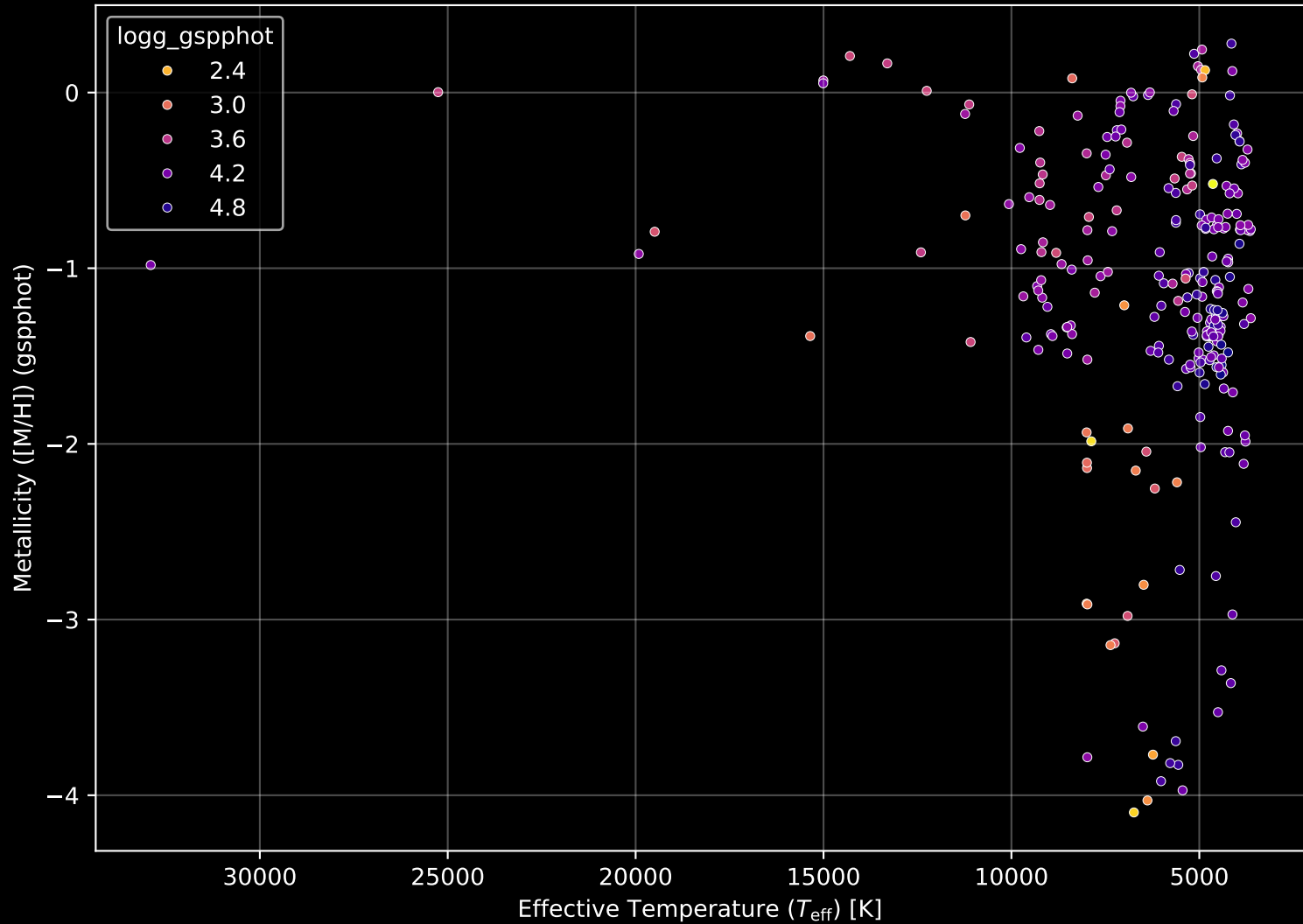
Gaia Cluster: [NGC_6611] Stellar Population Parameters (n= 278)
