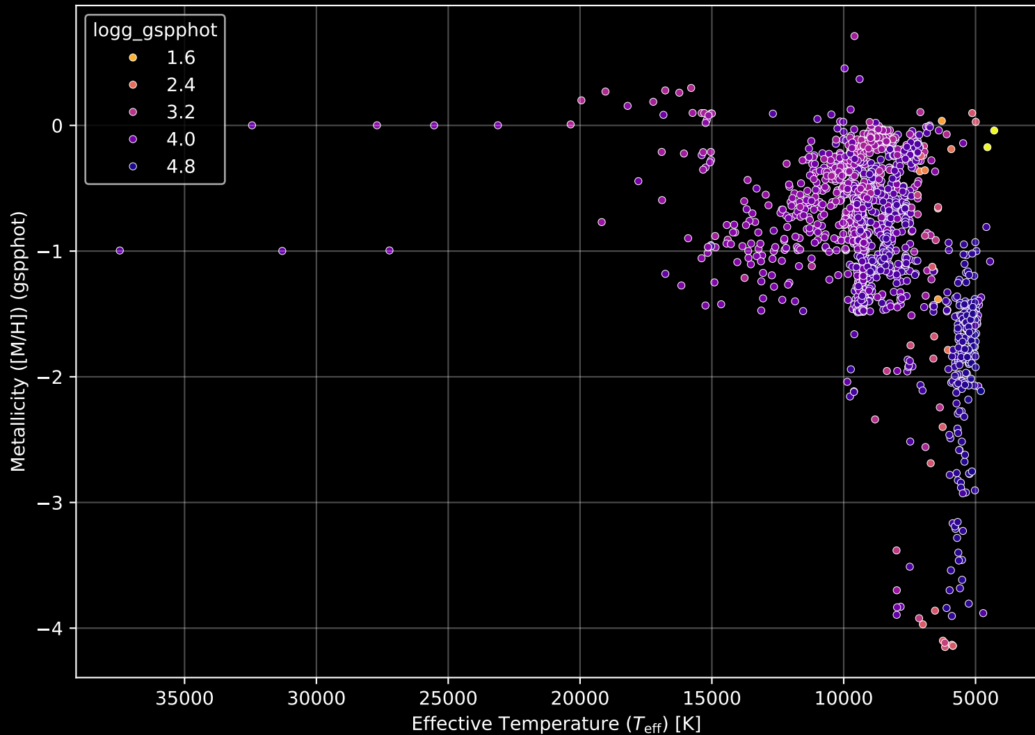
Gaia Cluster: [NGC_663] Stellar Population Parameters (n= 1494)
