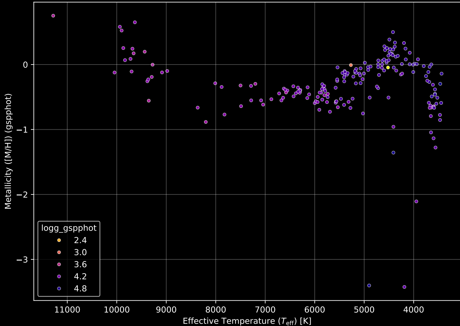
Gaia Cluster: [NGC_6633] Stellar Population Parameters (n= 192)
