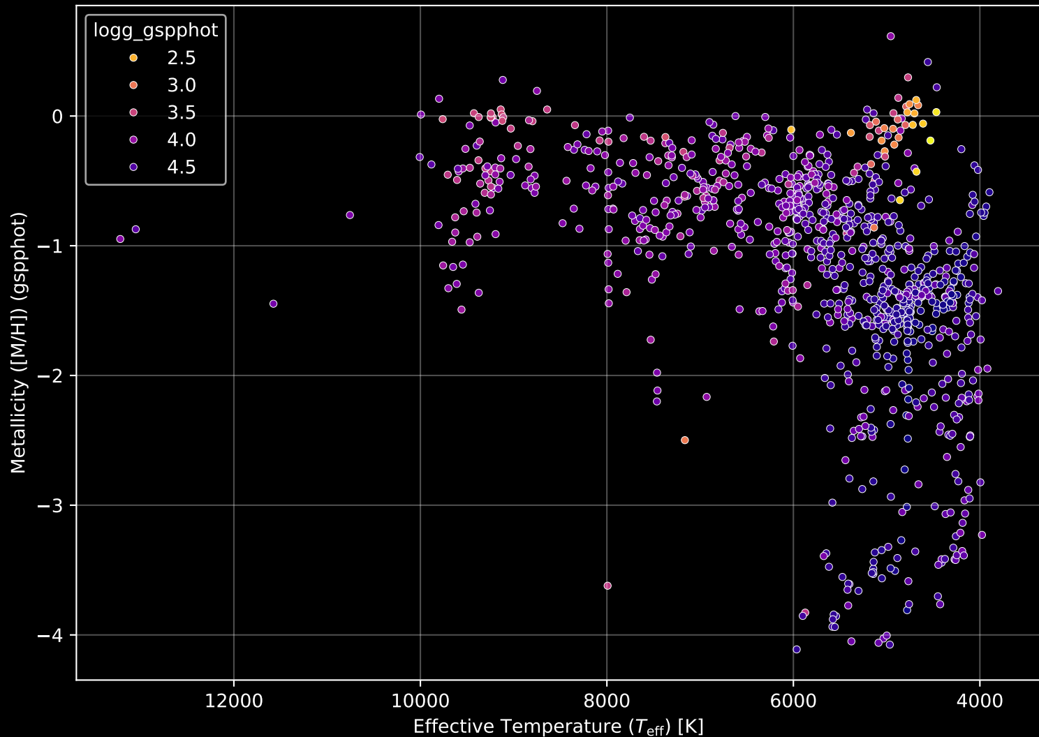
Gaia Cluster: [NGC_6645] Stellar Population Parameters (n= 988)
