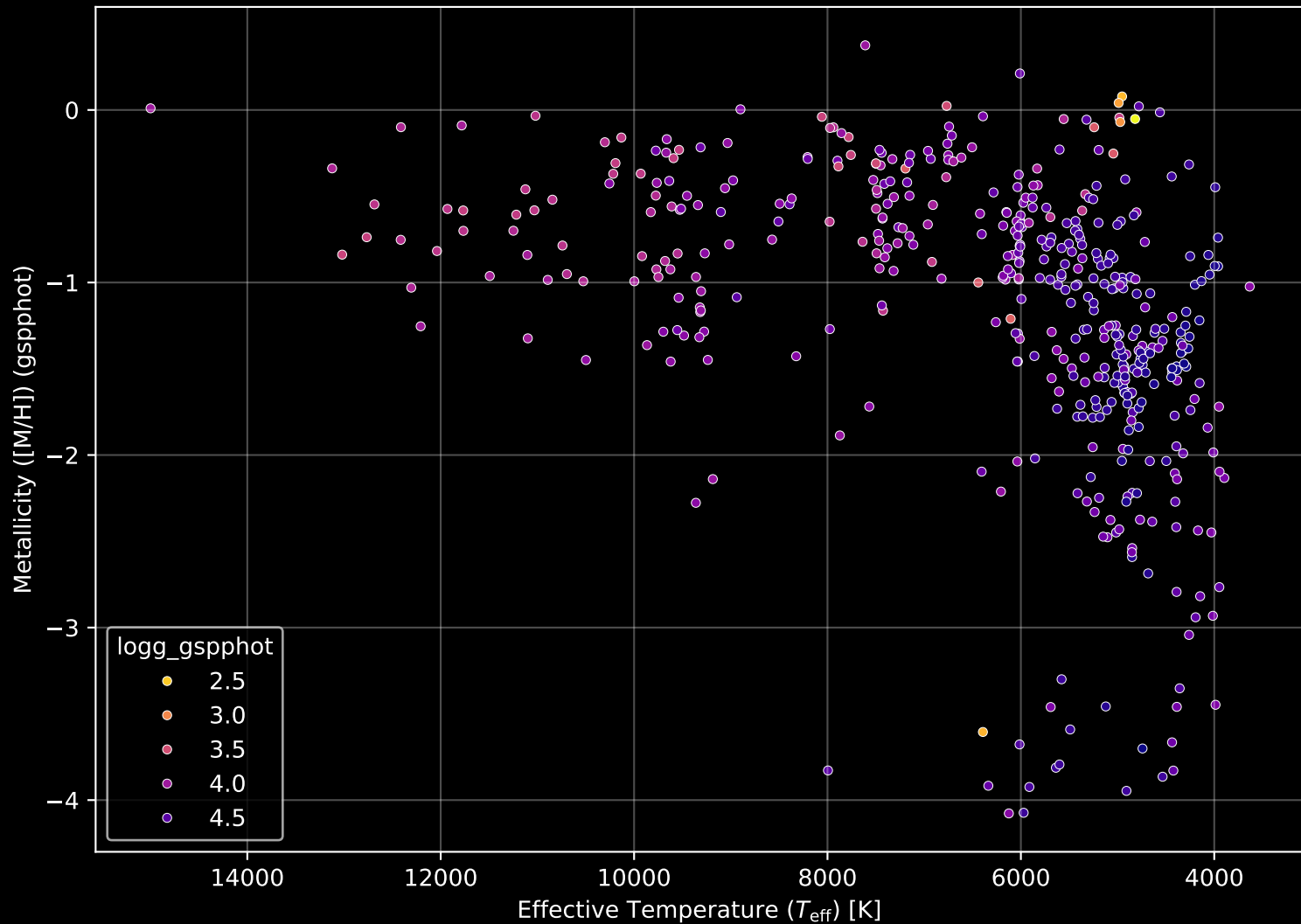
Gaia Cluster: [NGC_6694] Stellar Population Parameters (n= 473)
