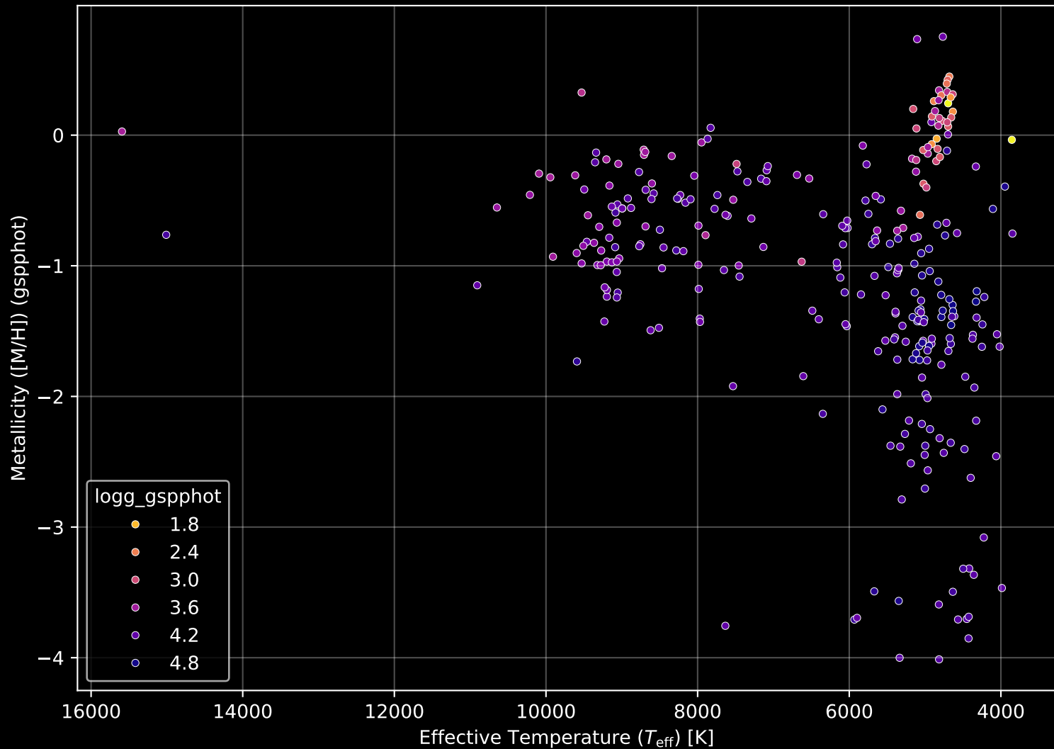
Gaia Cluster: [NGC_6704] Stellar Population Parameters (n= 298)
