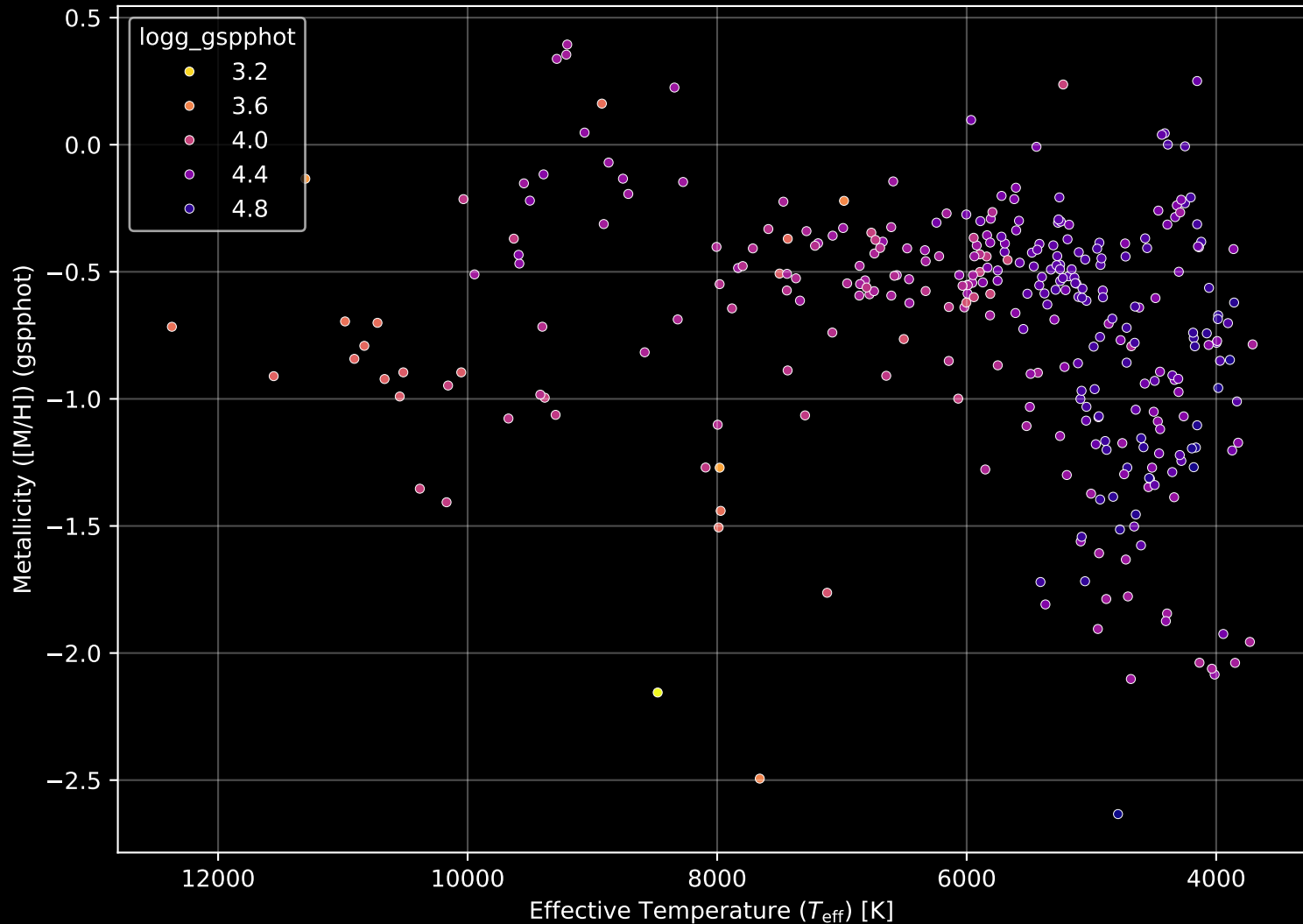
Gaia Cluster: [NGC_6709] Stellar Population Parameters (n= 321)
